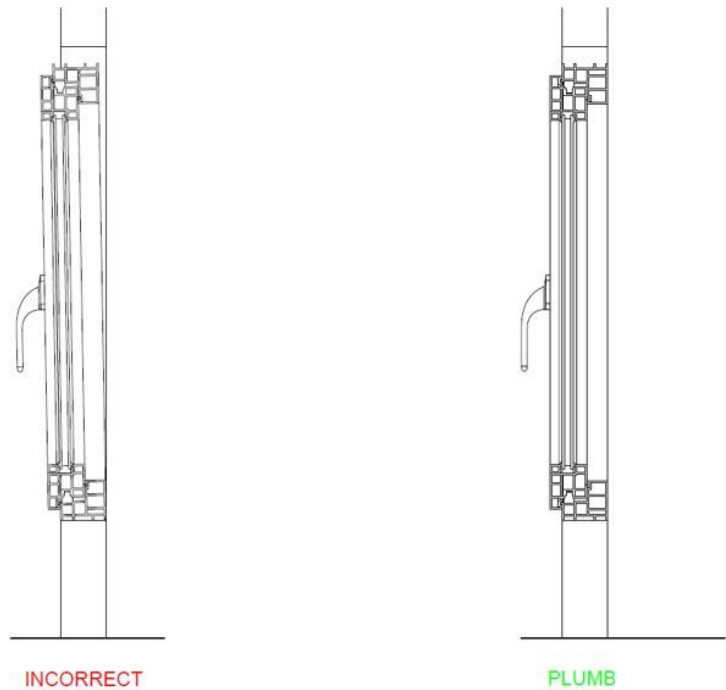
Fig. 6. Plumb:
