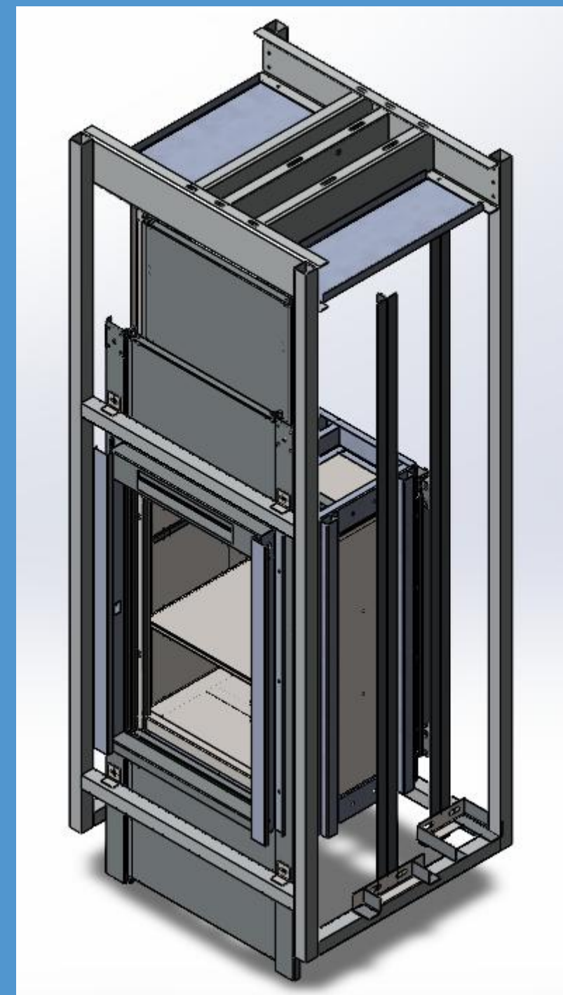
Кухонный, малый грузовой лифт, грузоподъемностью 60кг
