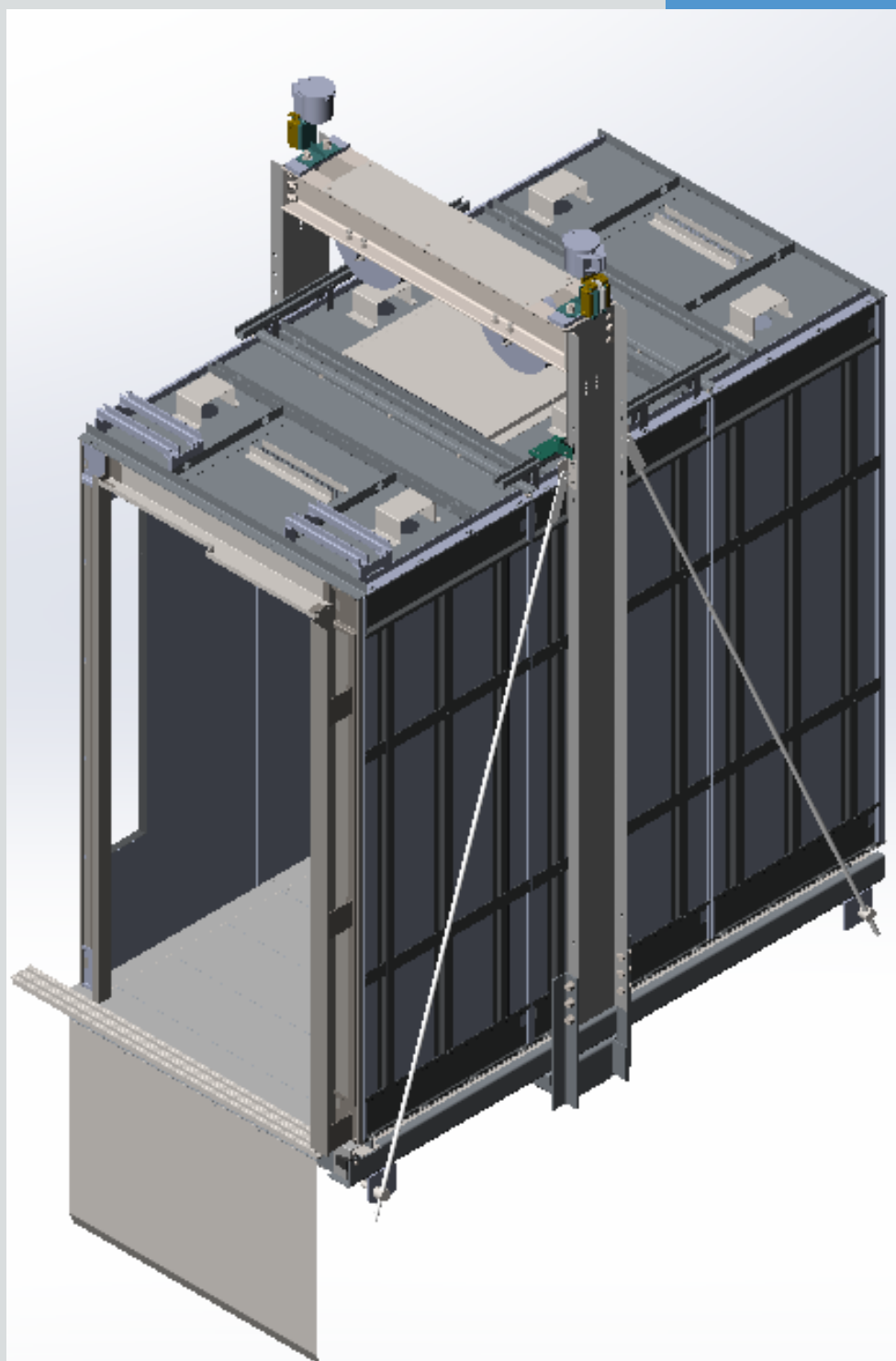
Грузопассажирский лифт (для больницы). Грузоподъемность 1000 кг.
