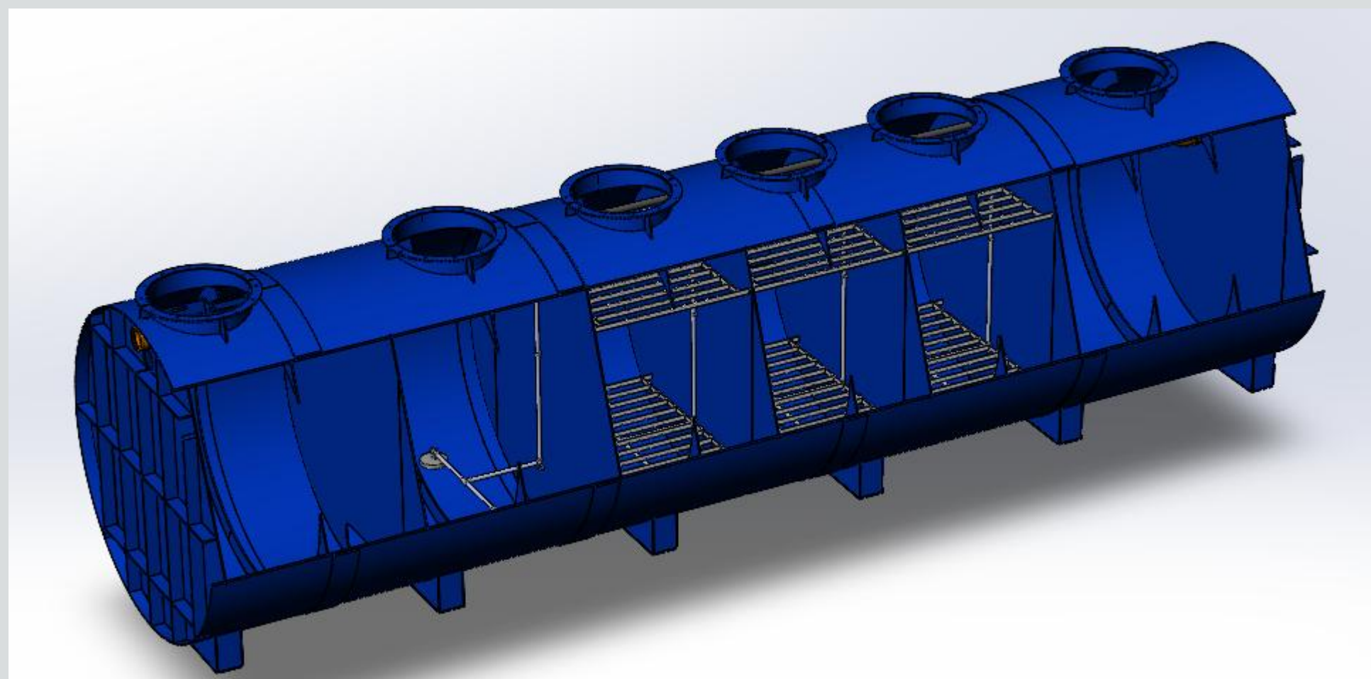
ЛЛОС цилиндрический горизонтальный, рассчитан на 150 чел. Полипропилен.
