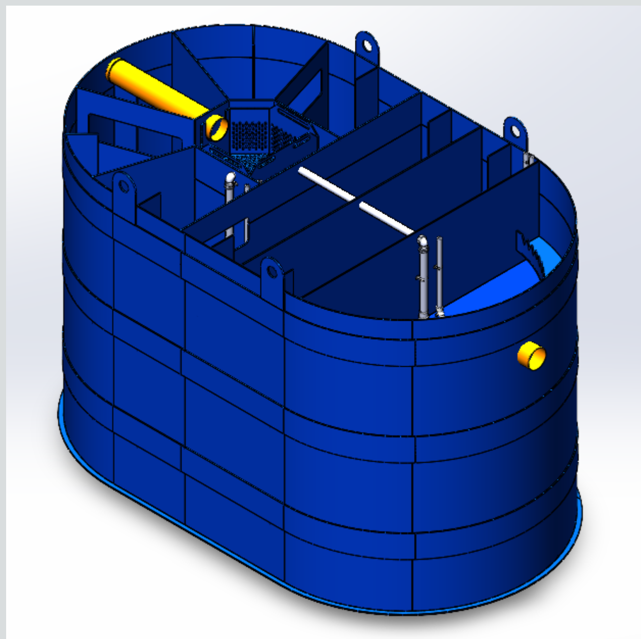
Биореактор. Локально очистные сооружения (ЛОС) рассчитан на 30 человек. Полипропилен.
