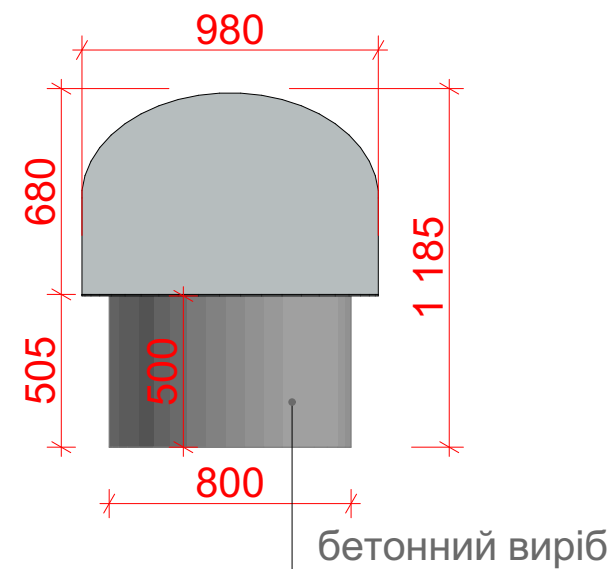
Вид спереду
