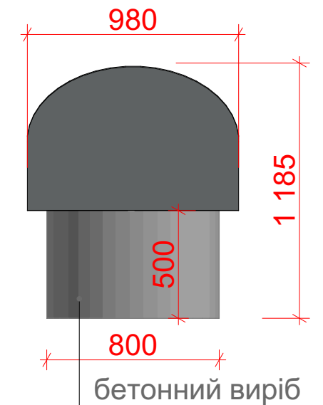
Вид ззаду
