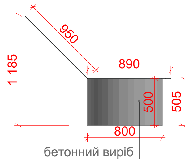
Вид зліва
