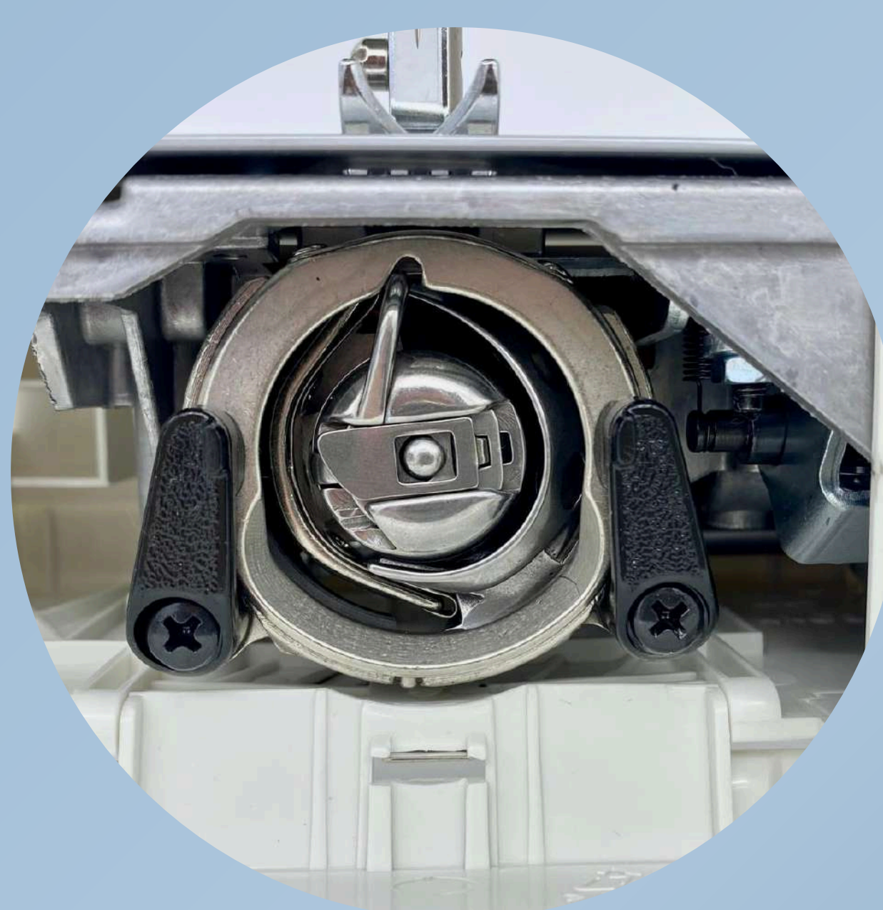
Вертикальный челнок
