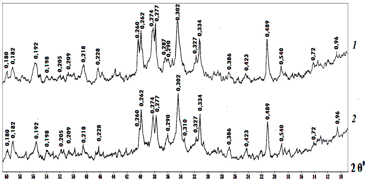
Рис. 3. Дифрактограма цементного каменю після тверднення протягом 2-х років:
