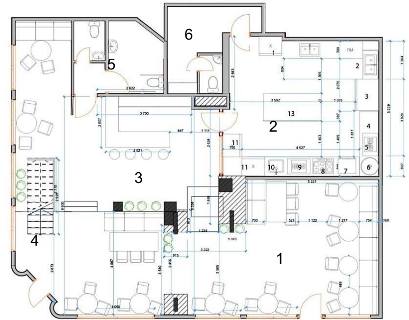
План кафе М 1:100
