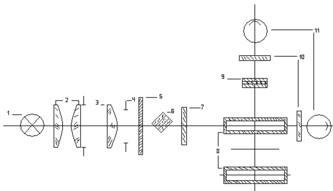
Рис. 19. Оптична схема фотометру ЛМФ - 72 М.1.
