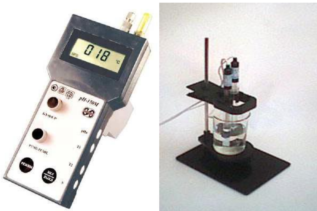
Рис. 22. рН-метр лабораторний рН-150М
