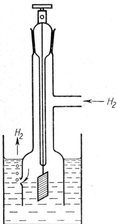
Рис. 23. Схема водневого електроду.
