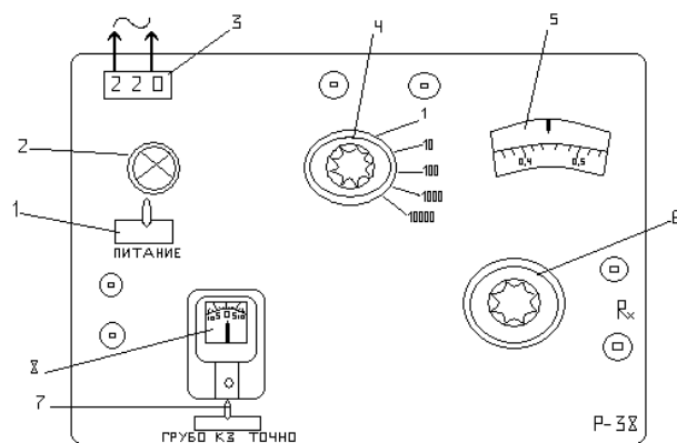
Рис. 29. Передня панель реохордного моста Р-38.
