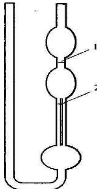
Рис.46. Капілярний віскозиметр Оствальда
