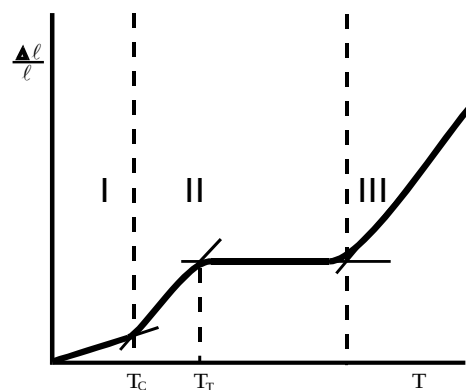
Рис. 43. Фазові стани ВМС: I – склоподібний; II – вискоеластичний; III – в'язкотекучий.
