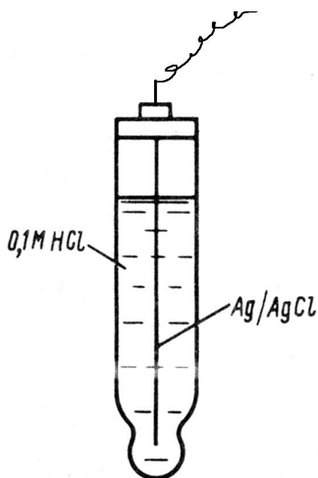
Рис. 24. Схема скляного електроду.
