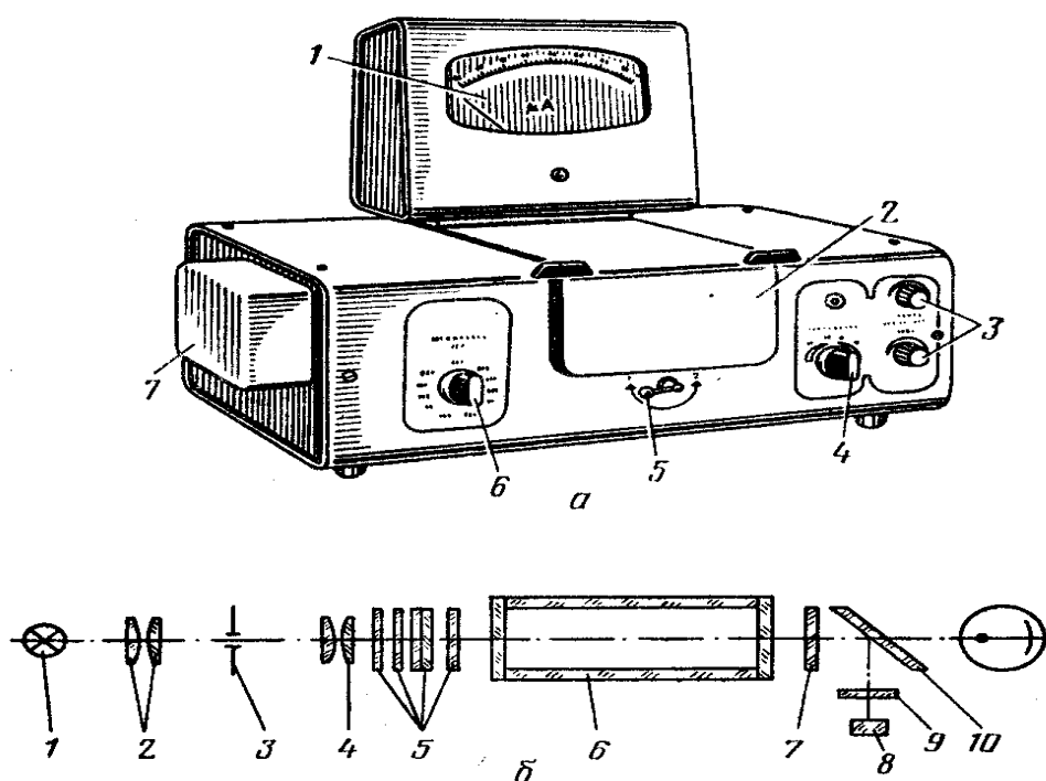
Рис. 10. Колориметр фотоелектричний концентраційний КФК-2.
