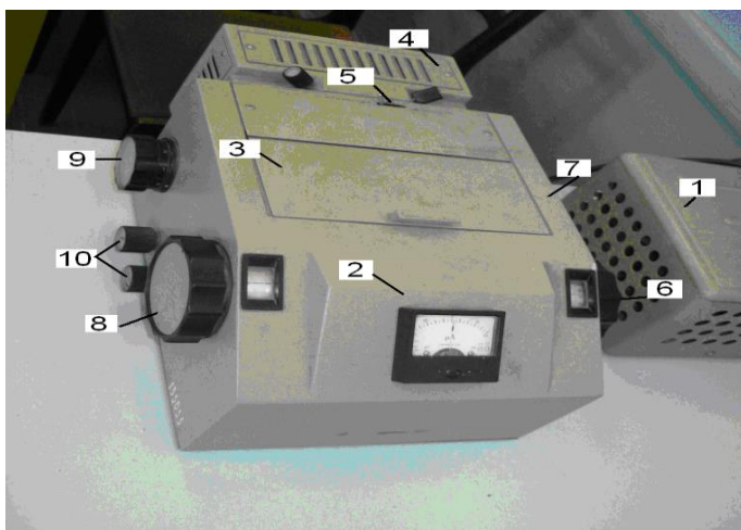
Рис. 39. Колориметр-нефелометр ФЭК-56М
