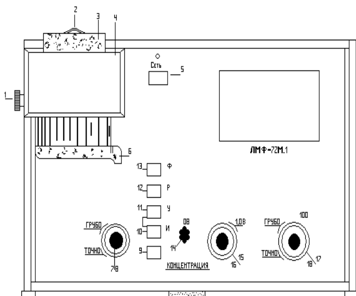
Рис. 18. Загальний вигляд фотометра ЛМФ 72 М.1
