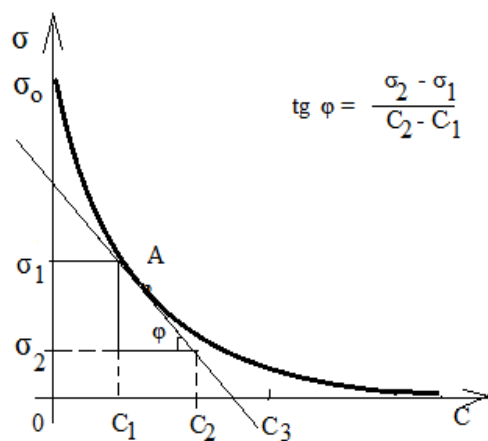
Рис. 31. Ізотера поверхневого натягу
