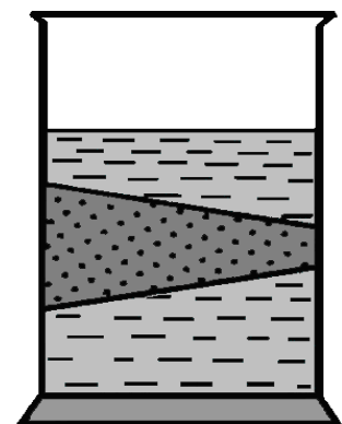
Рис. 37. Розсіювання світла колоїдними частинками (конус Тіндаля)
