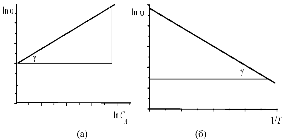
Рис. 4. Графічні залежності для визначення порядку реакції (а) та енергії активації (б).
