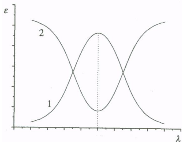
Рис. 9. Правило вибору світлофільтра: 1 - спектр поглинання забарвленої сполуки; 2 - спектр поглинання світлофільтра.
