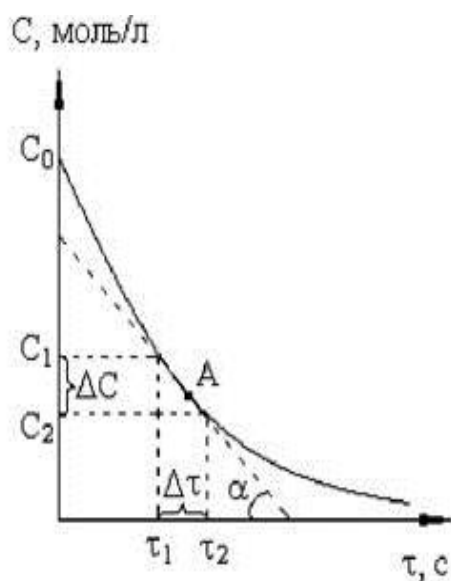
Рис. 3. Зміна концентрації речовини з часом реакції.
