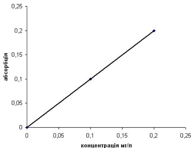
Рис. 12. Калібрувальний графік для визначення концентрації забарвленого розчину.
