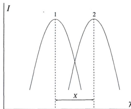
Рис. 14. Дзеркальна симетрія спектрів родамину в ацетоні:
