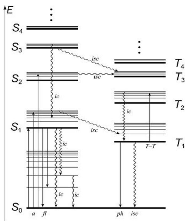
Рис. 15. Схема Яблонського
