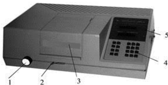
Рис. 11. Фотометр фотоелектричний КФК-3: 1: ручка настройки довжин хвиль; 2: перемикач кюветного відділення; 3: кришка кюветного відділення; 4: клавіатура управління; 5: цифрове табло
