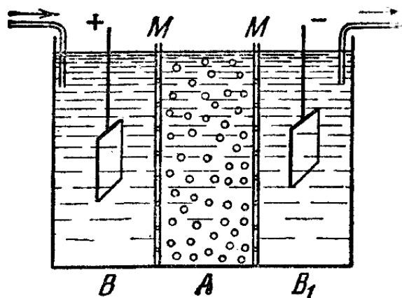
Рис. 34. Схема електродіалізатора.
