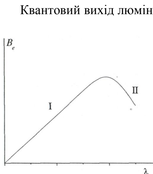
Рис. 16. Залежність квантового виходу люмінесценції від довжини хвилі збуджуючого світла
