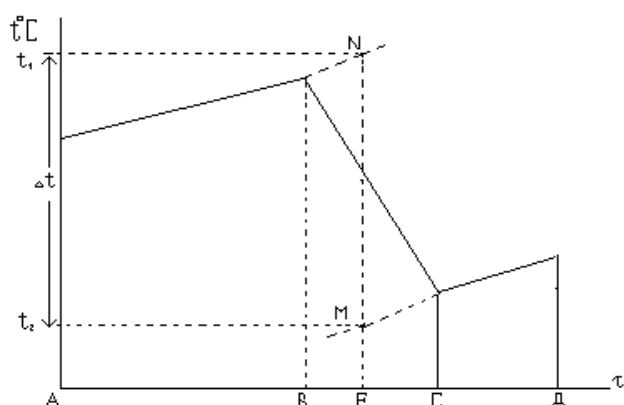
Рис. 2. Зміна температури при розчиненні речовини (АВ – попередній період, ВС – головний, СД – заключний)
