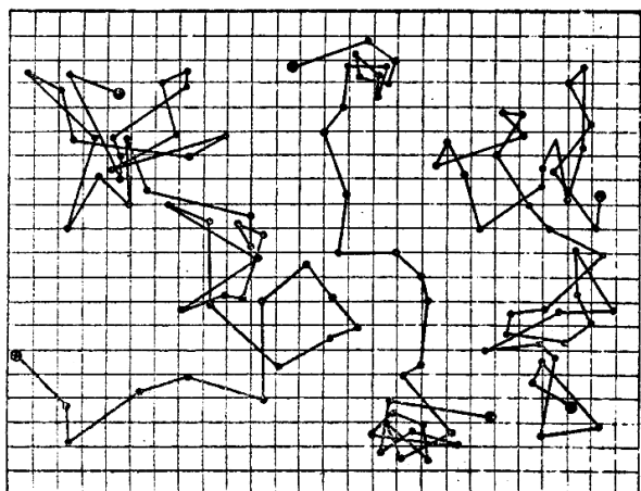
Рис. 36. Броунівський рух частинок.
