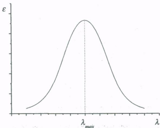
Рис. 7. Електронний спектр поглинання забарвленої сполуки в розчині.
