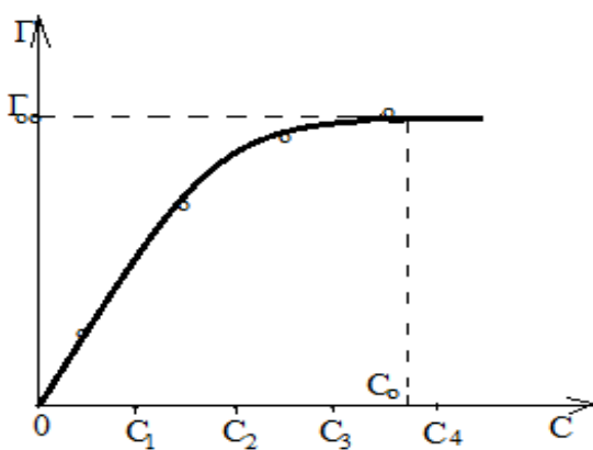
Рис. 30. Ізотерма адсорбції
