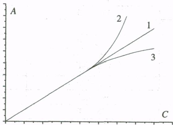
Рис. 8. Відхилення від основного закону світлопоглинання: 1: лінійна залежність оптичної густини ( A ) від концентрації ( C ); 2: позитивне відхилення; 3: негативне
