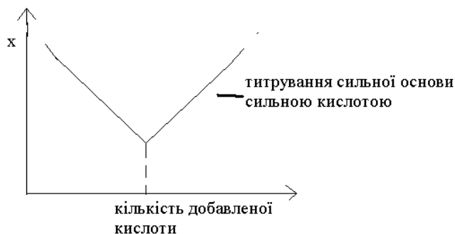
Рис. 27. Крива кондуктометричного титрування
