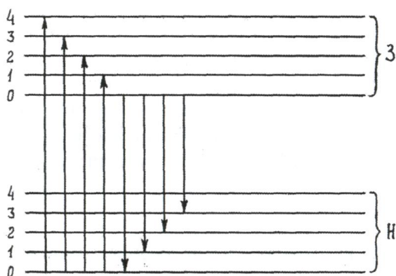
Рис. 13. Схема процесів виникнення світіння молекул.
