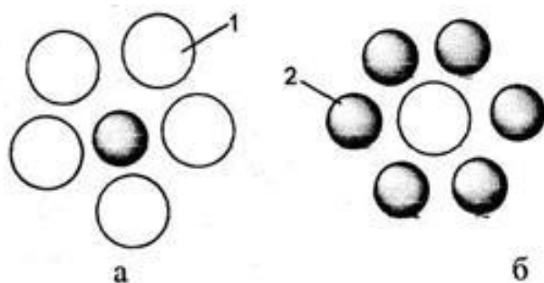
Рис. 35. Явище "захисту" (а) і астабілізації (б) колоїдної частинки; 1-поверхнево-активна речовина; 2 – золь
