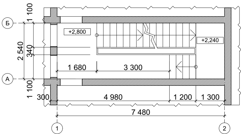
План на відм. 2,800
