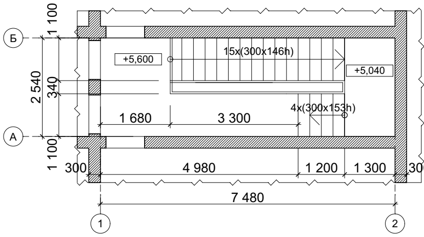
План на відм. 5,600
