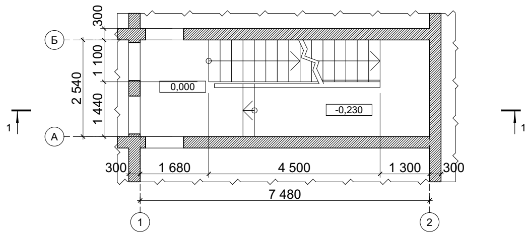
План на відм. 0,000
