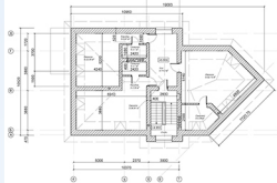
План мансардного поверху на відм. +6.600
