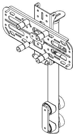
11. Стойка монитора
