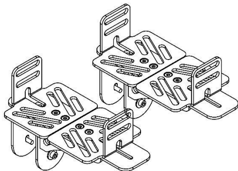
7. Полки крепления проводов
