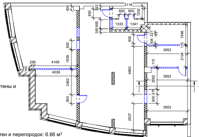
План монтажа стен и перегородок М 1:100
