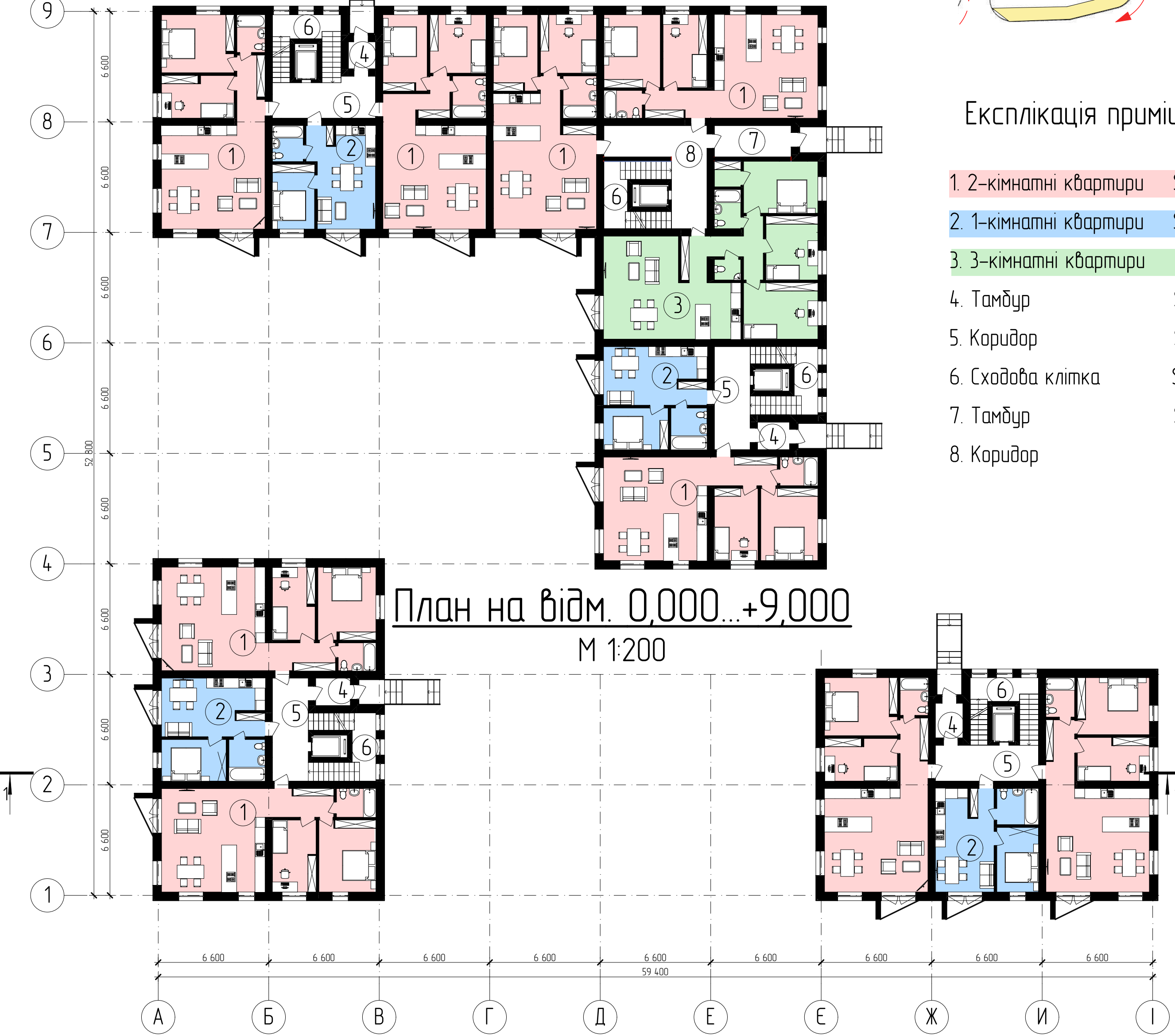
План на відм. 0,000...+12,000 М 1:200
