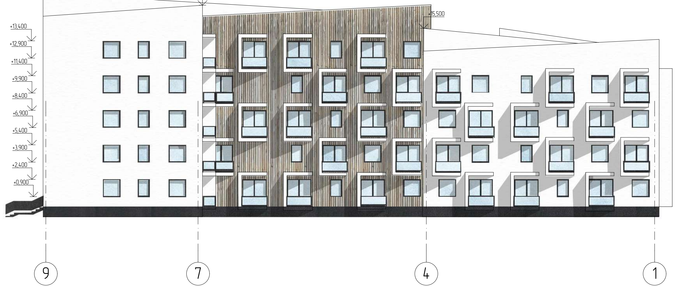
Фасад 9-1 М 1:200
