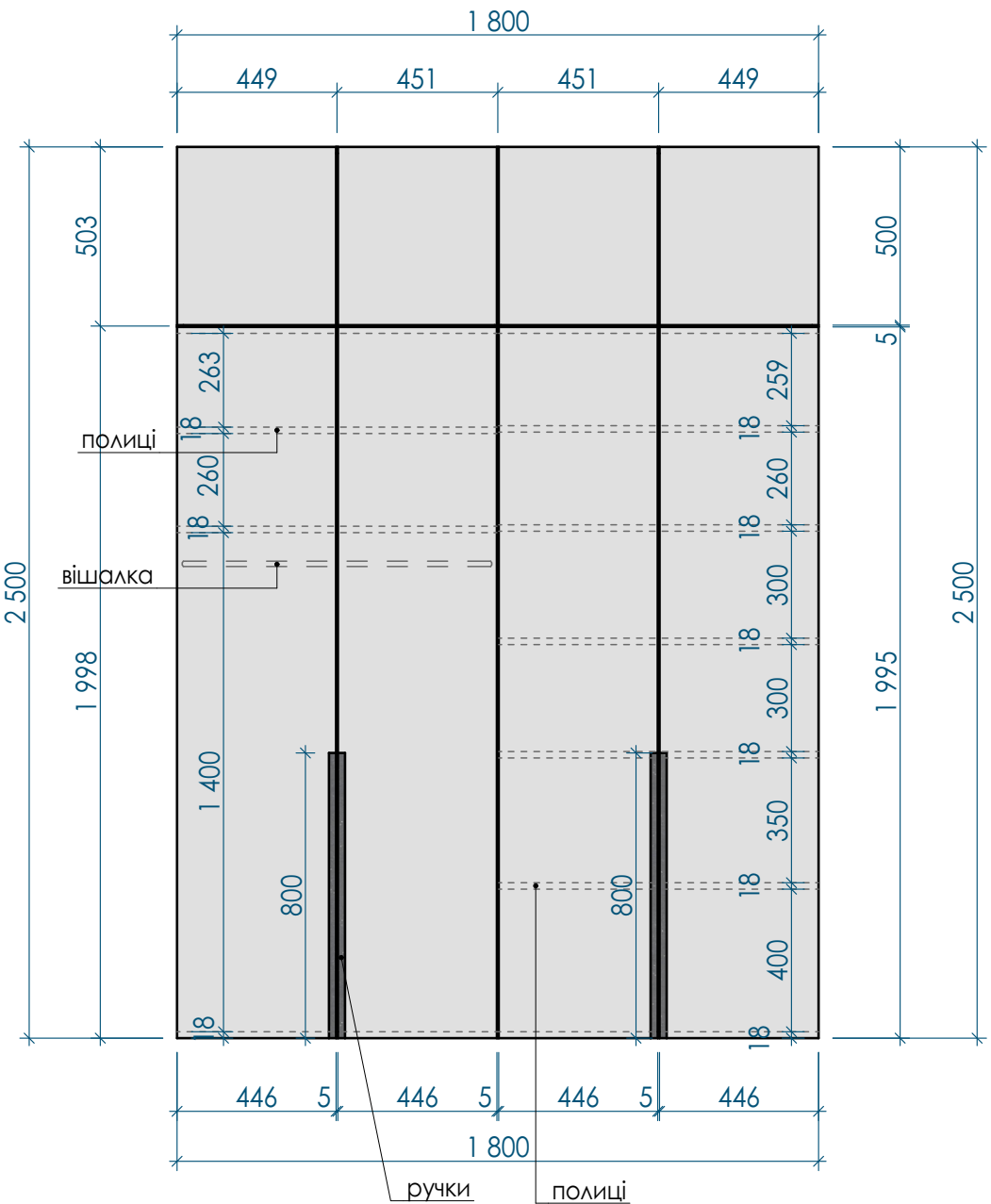
Вигляд спереду
