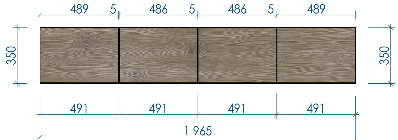
Вигляд спереду
