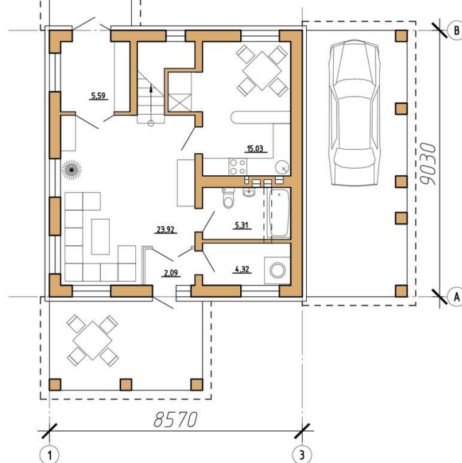
План 1-ого поверху
