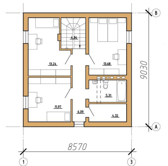
План 2-ого поверху
