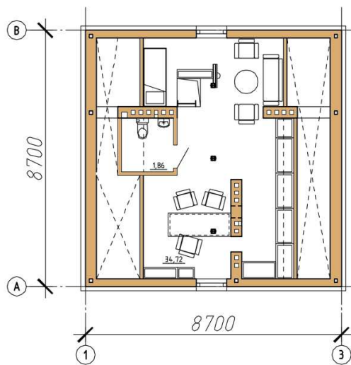
План мансардного поверху
