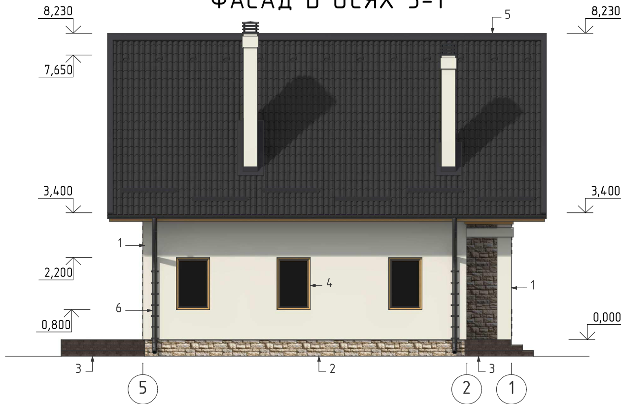
ФАСАД В ОСЯХ 5-1
