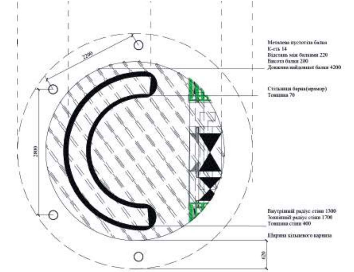
План альтанки
