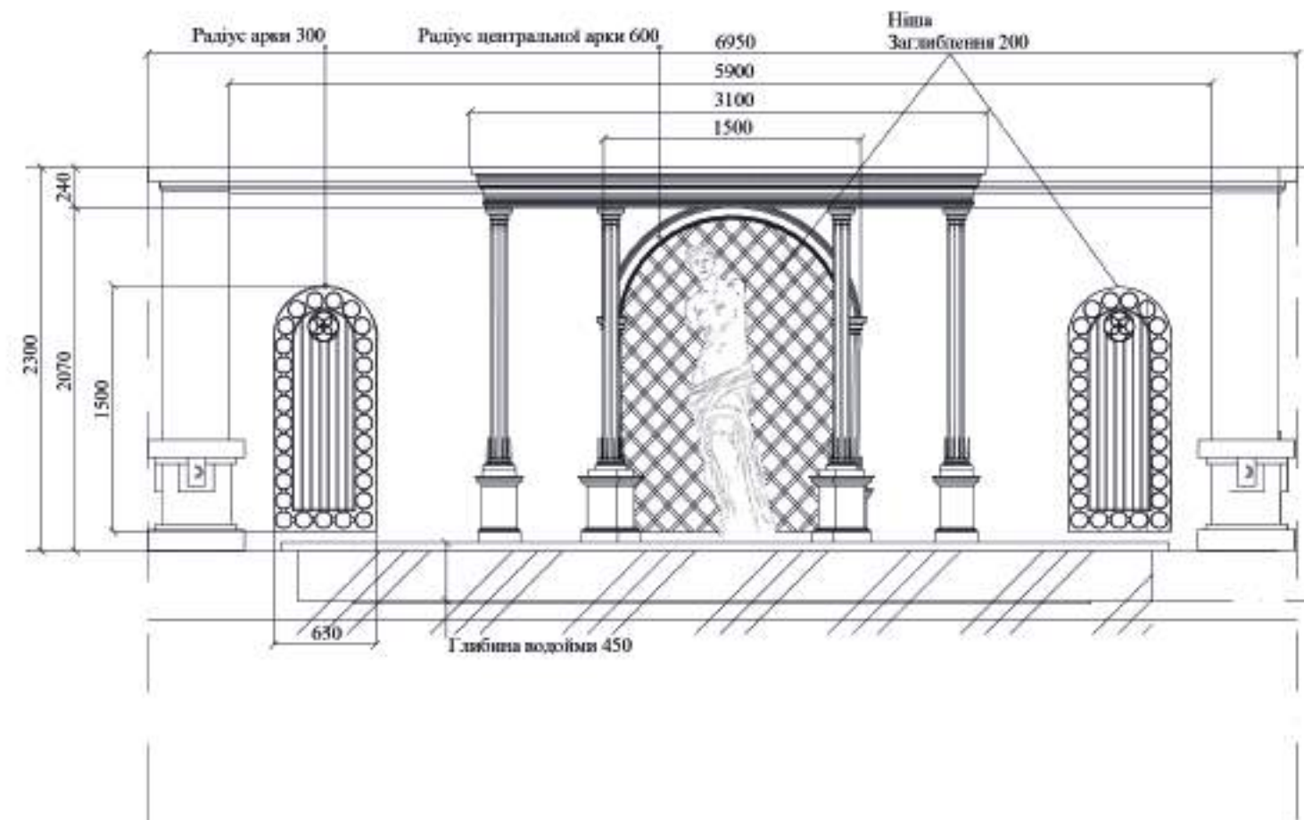
Розріз А
