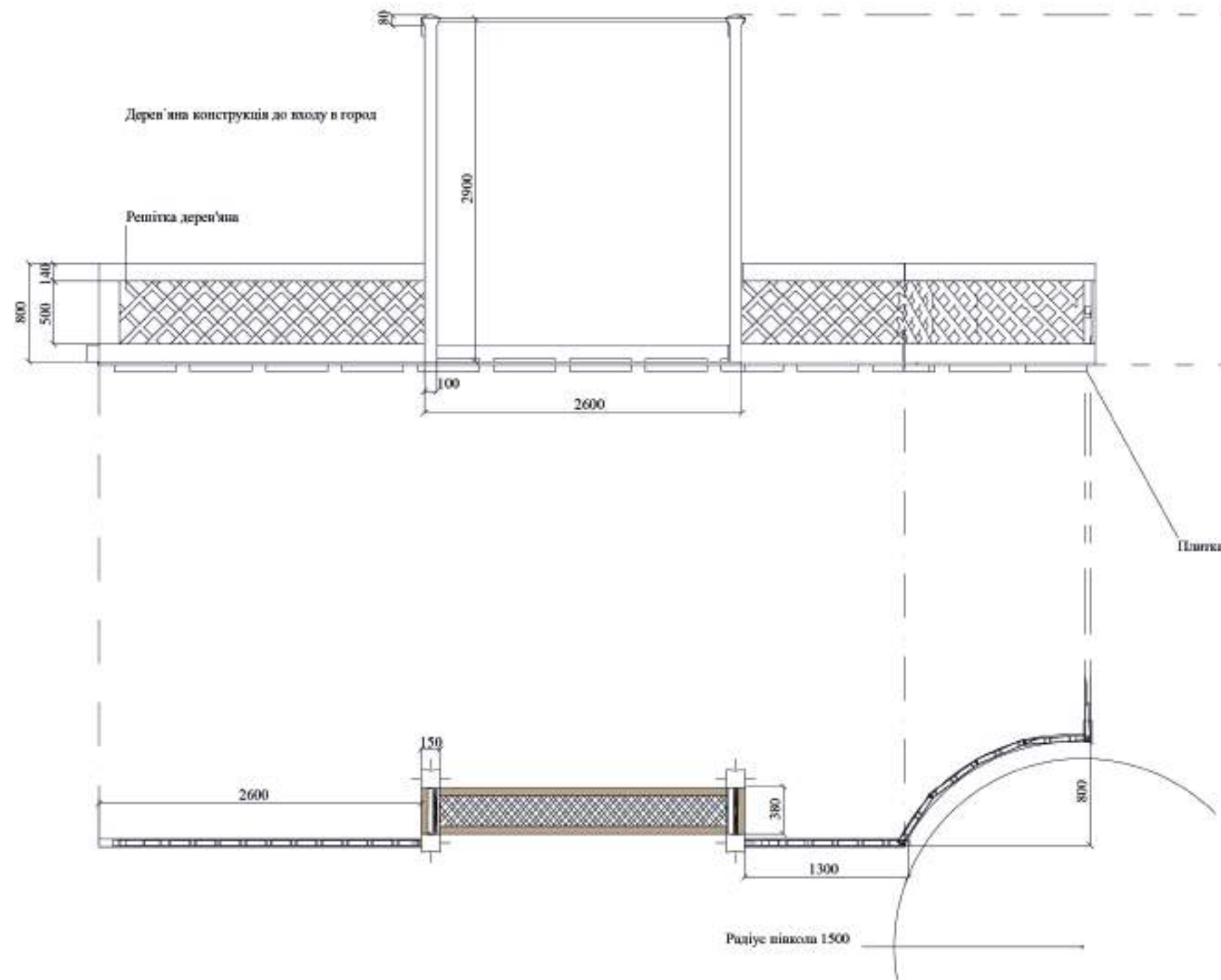
Розріз А
