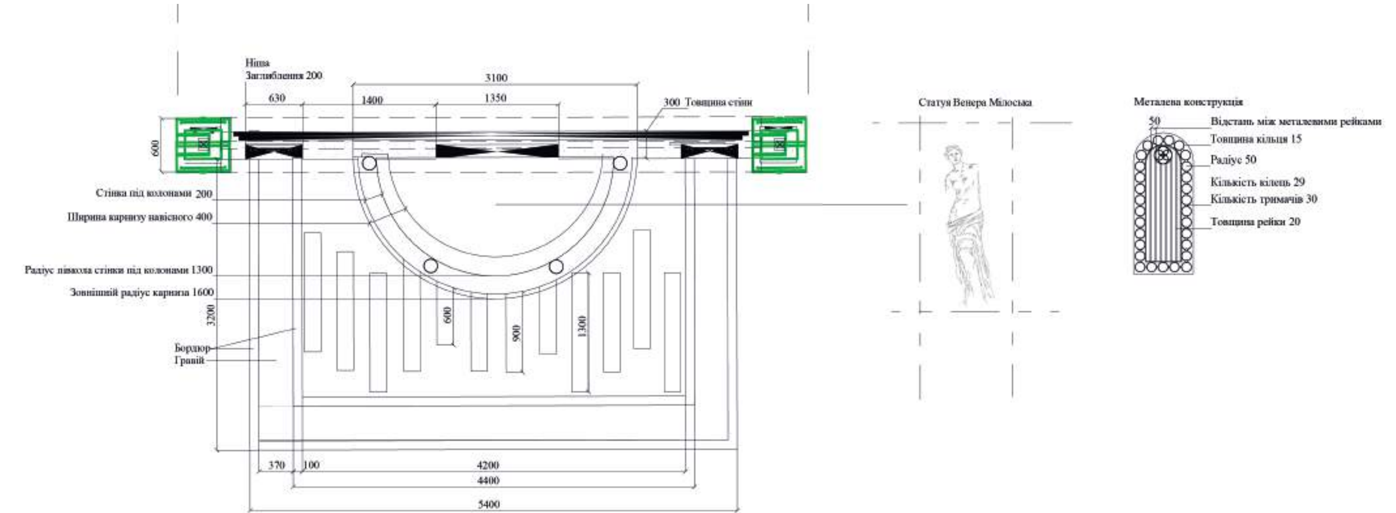
Розріз Б
