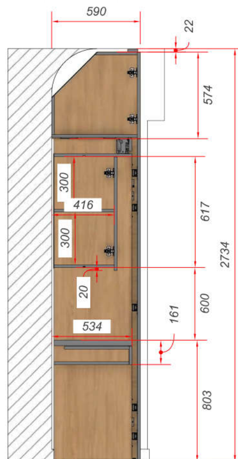
Разрез В
