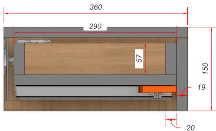
Вид слева (разрез)
