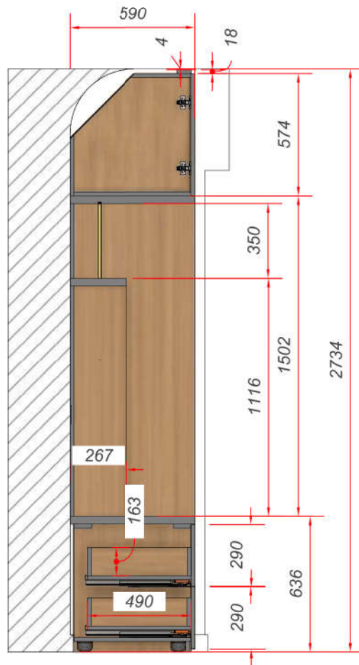
Разрез Б
