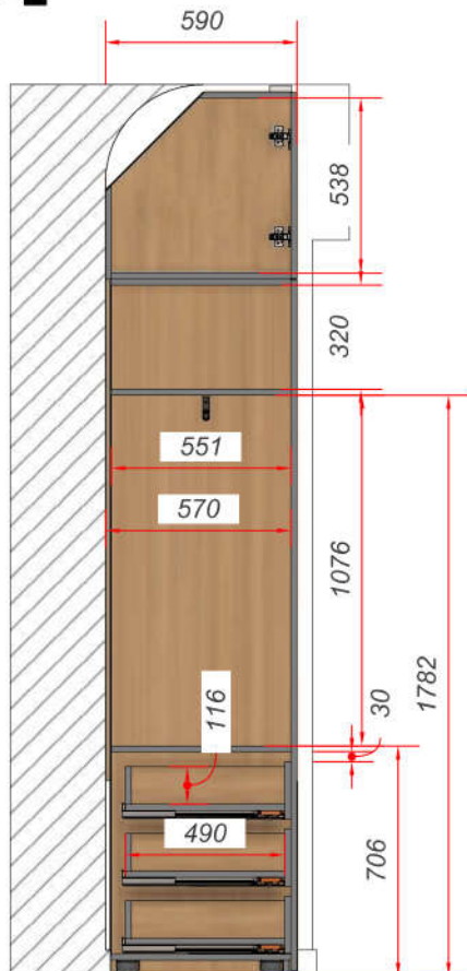
Разрез А
