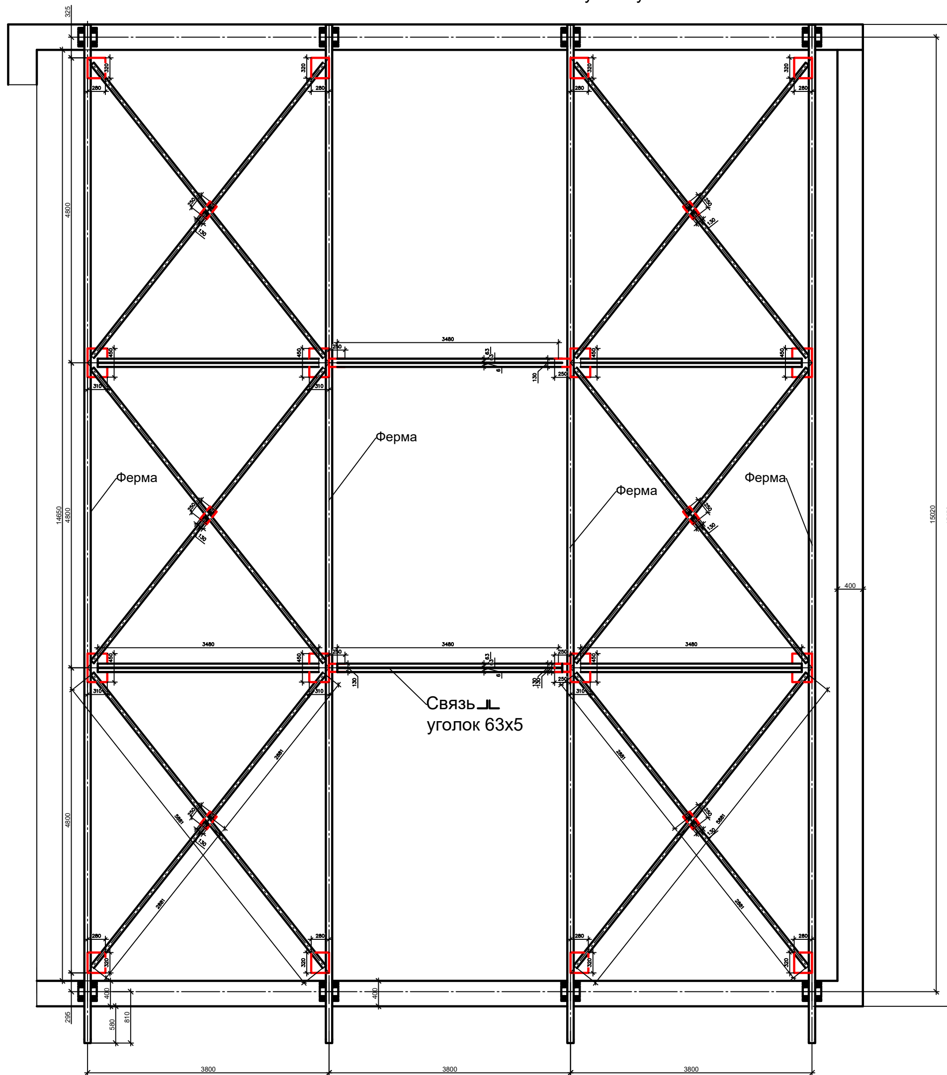
План связей по нижнему поясу
