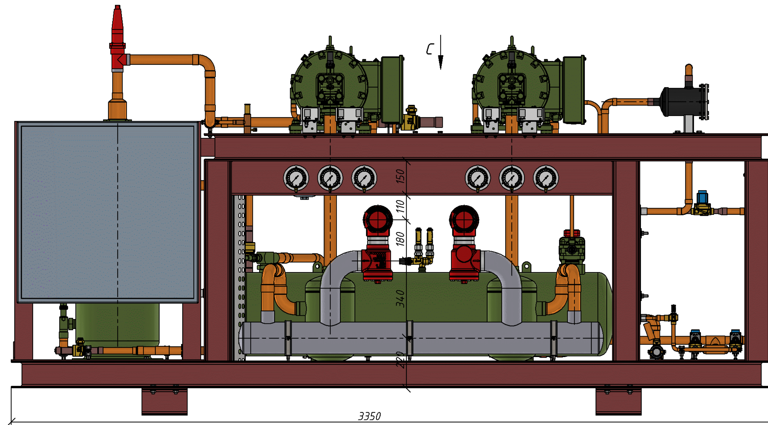
A-A (1:10)
