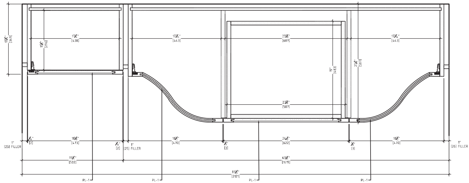
1 PLAN SECTION SCALE: 1-1/2"=1'-0"
