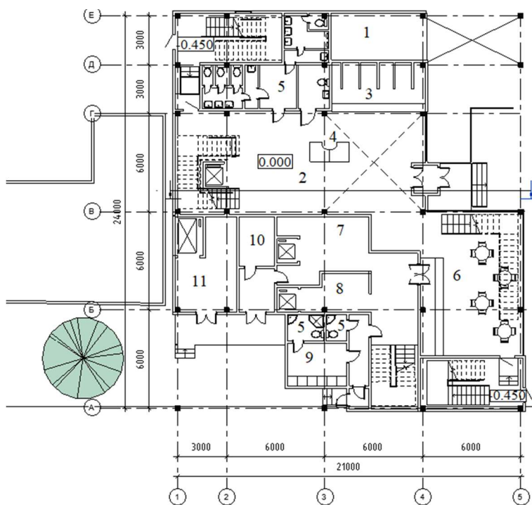
Експлікація до плану на відмітці 0.000
