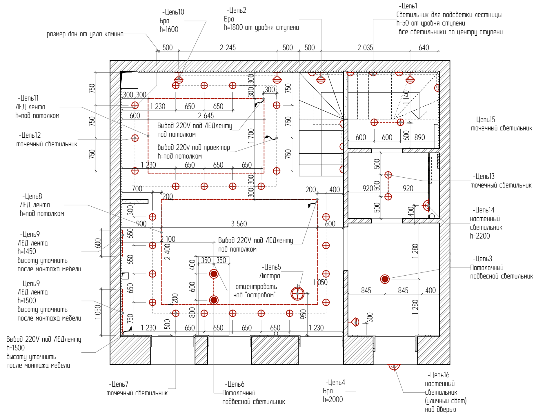
Ведомость осветительных приборов, 1 этаж
