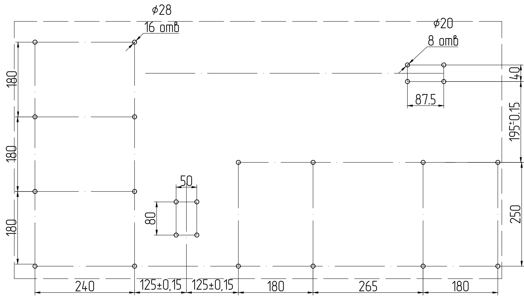
Схема розташування монтажних отворів
