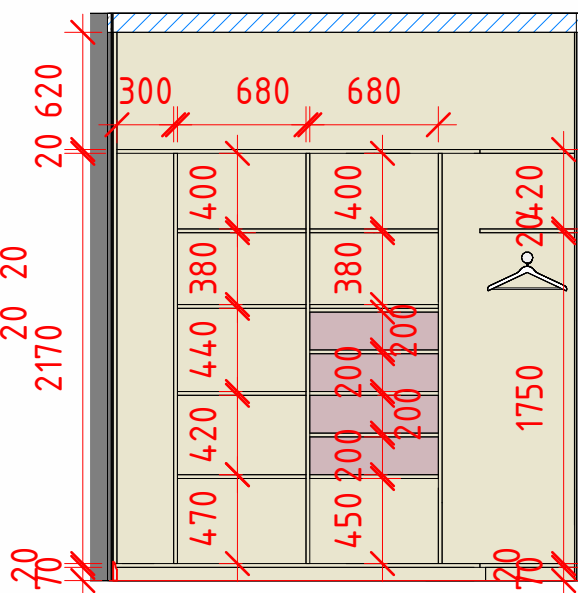
Гардероб у спальні 1-1 1:40
