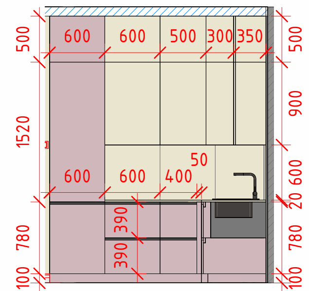
Кухня (вид на холодильник) 1:40
