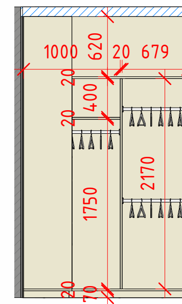
Гардероб у спальні 1-2 1: 40
