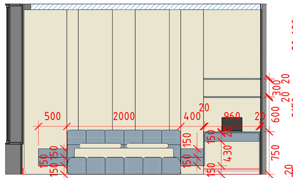
Тумби та стіл (спальня) 1:40
