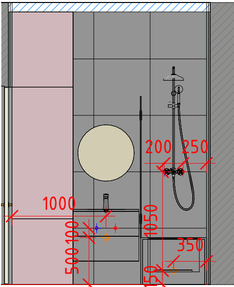
Ванна кімната (умивальник) 1: 40
