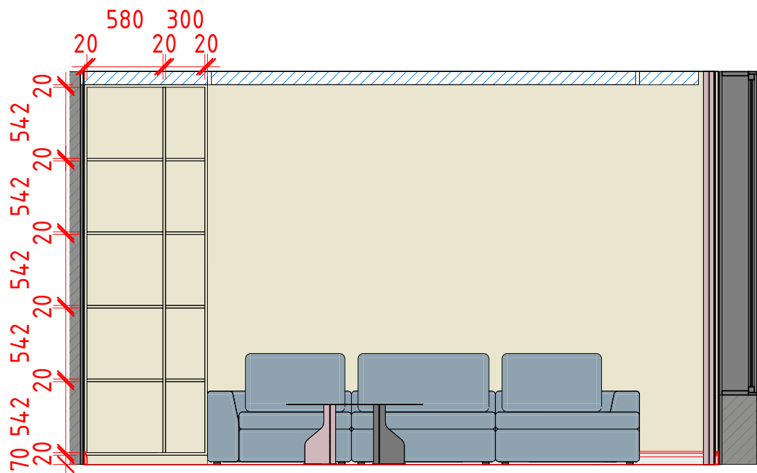
Шафа (вітальня/ внутрішня частина) 1: 40
