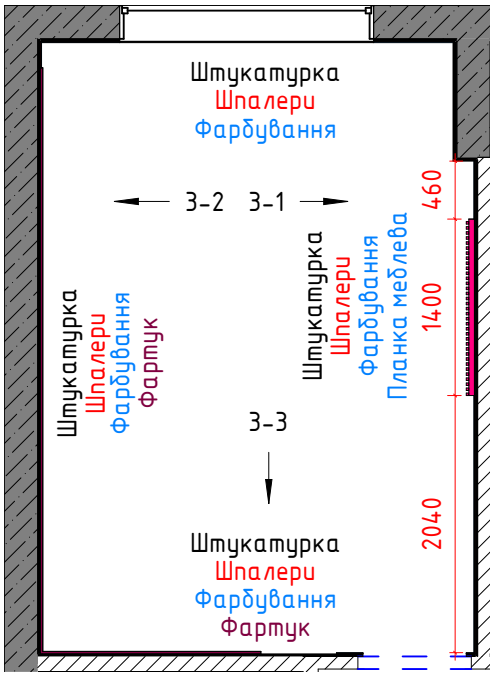
План обробки (кухня)
