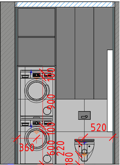
С/В (прал. та суш. маш.) 1: 40
