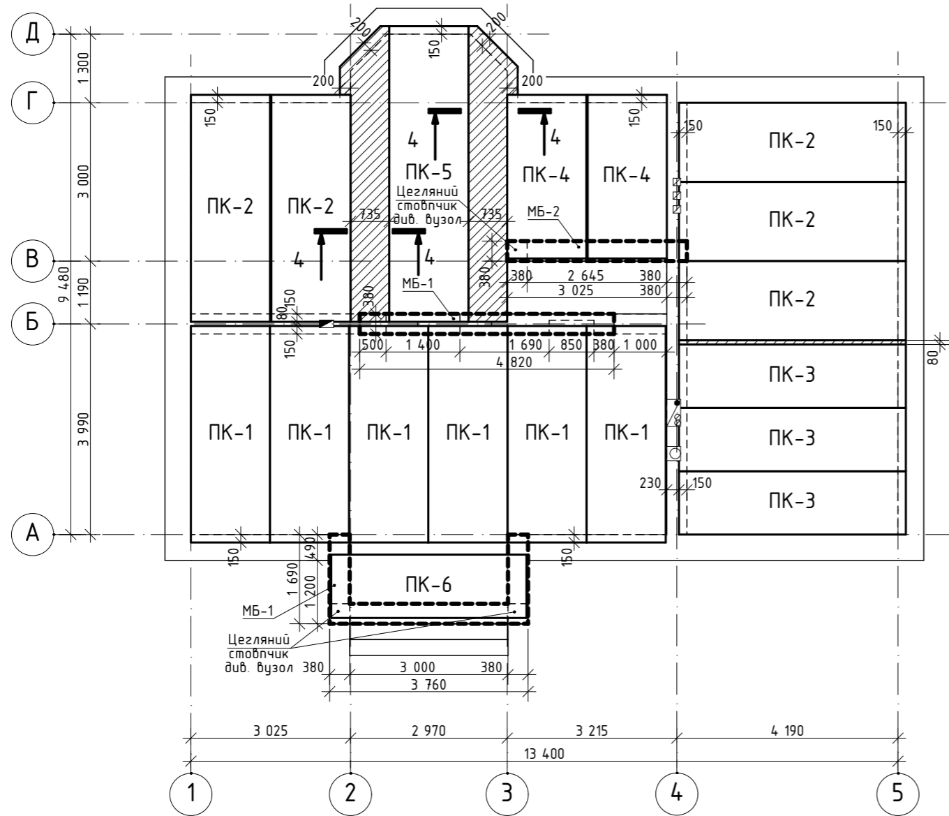
План перекриття низ на позн. +2,800
