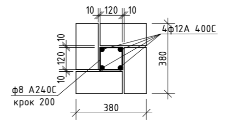
Армування цегляного стовпчику
