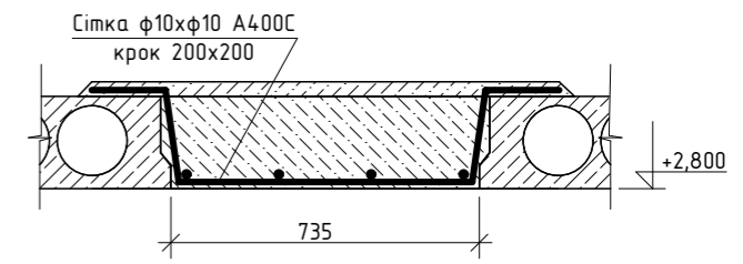
Розріз 4-4
