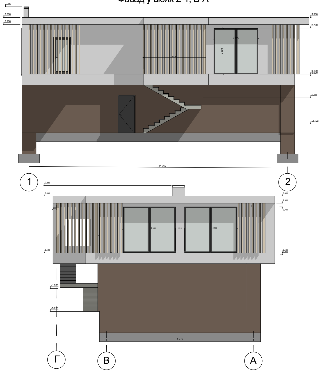
Фасад у вісях 2-1, В-А
