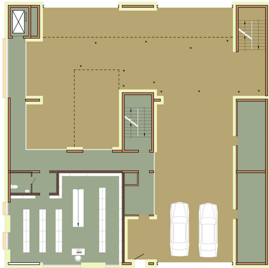
План 1 этажа
