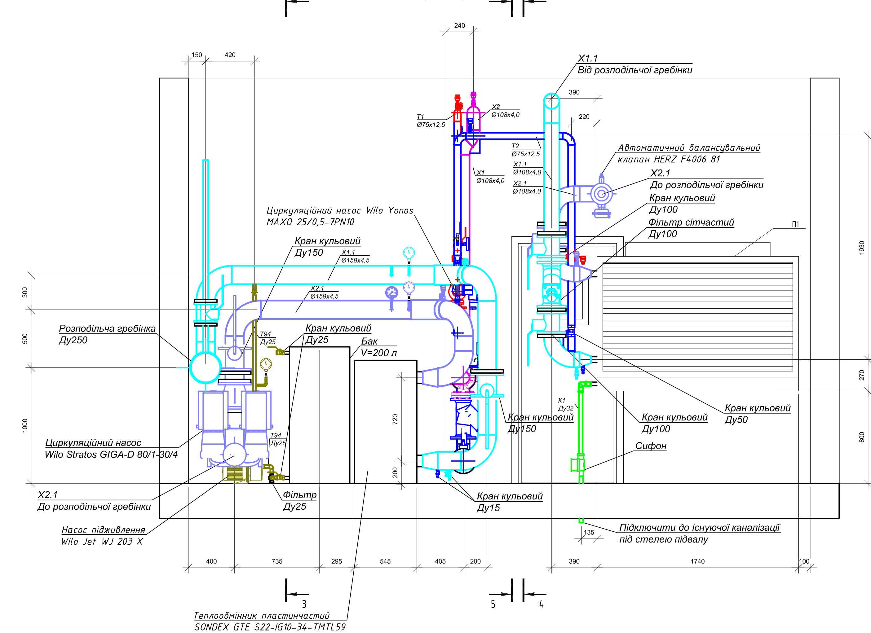
Розріз 2-2 (М1:20)
