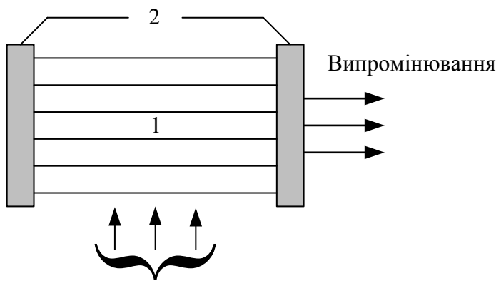
Струм накачування 1 – активне середовище; 2 – дзеркала резонатора
