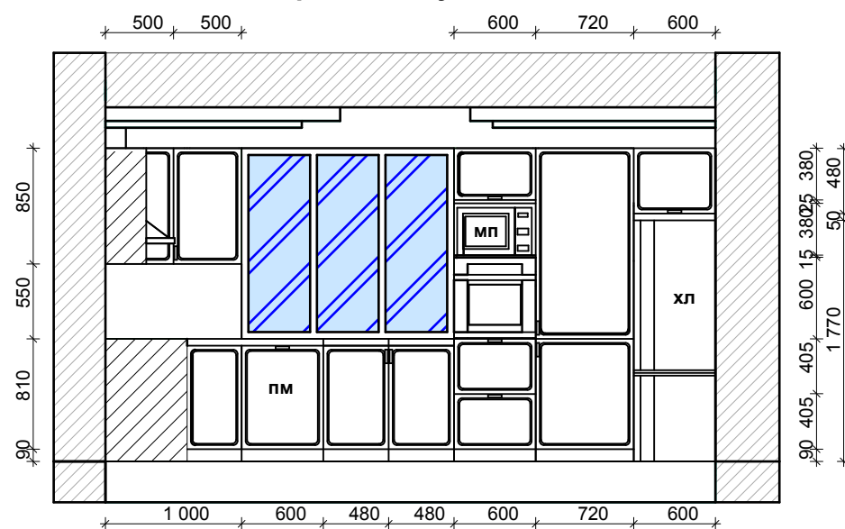
Розгортка стін кухні по осях 2-1 М 1:50
