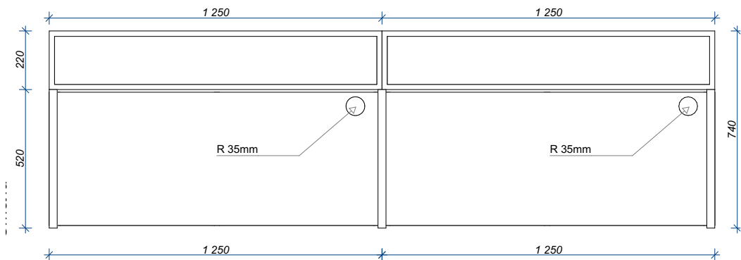
Вид зверху
