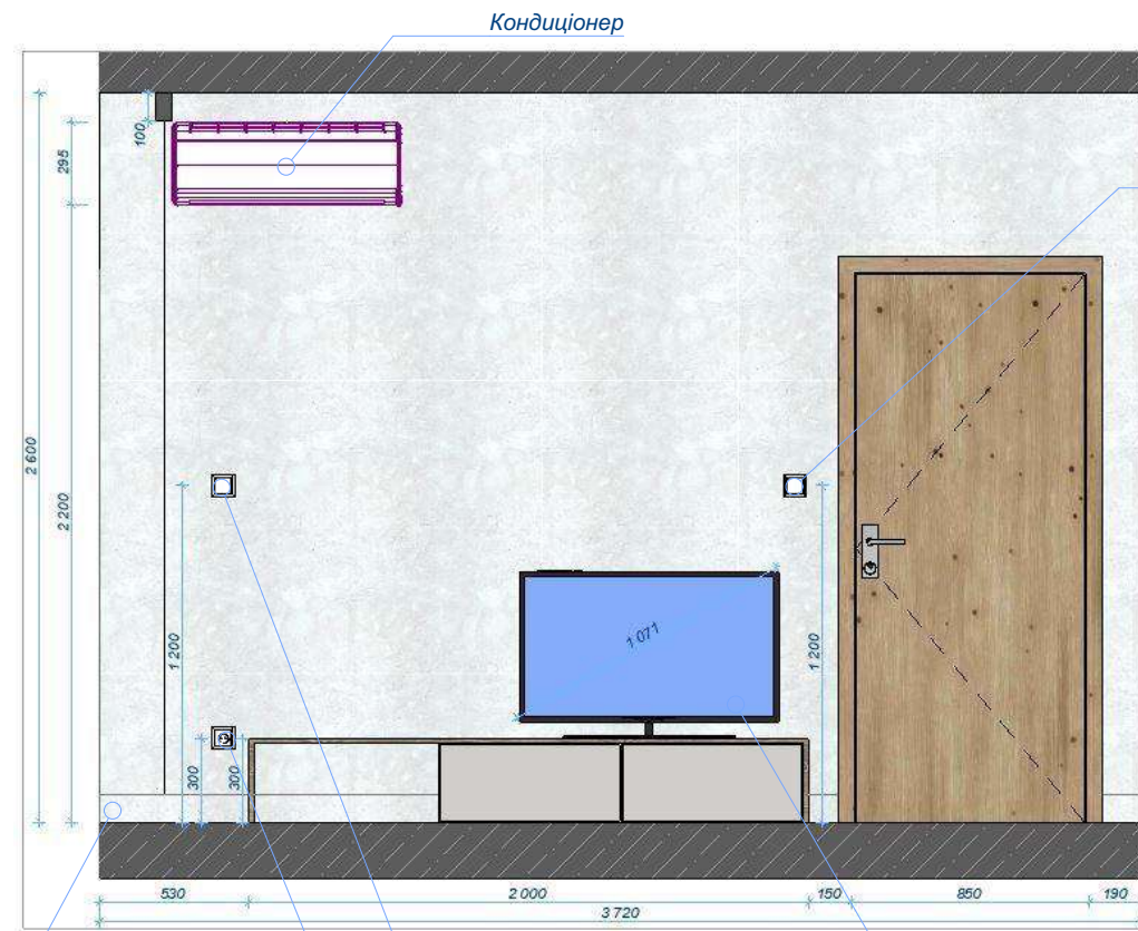
2 Розетка Одноклавішний вимикач Tv 1:30
