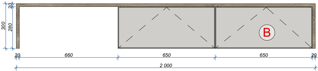
Вид спереди
