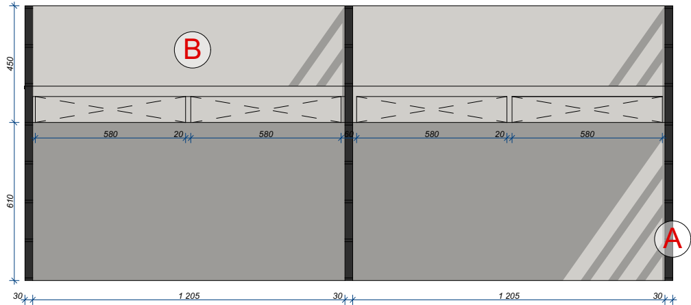
Вид спереди
