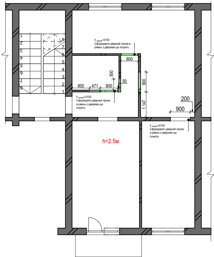
План монтажу М1:100
