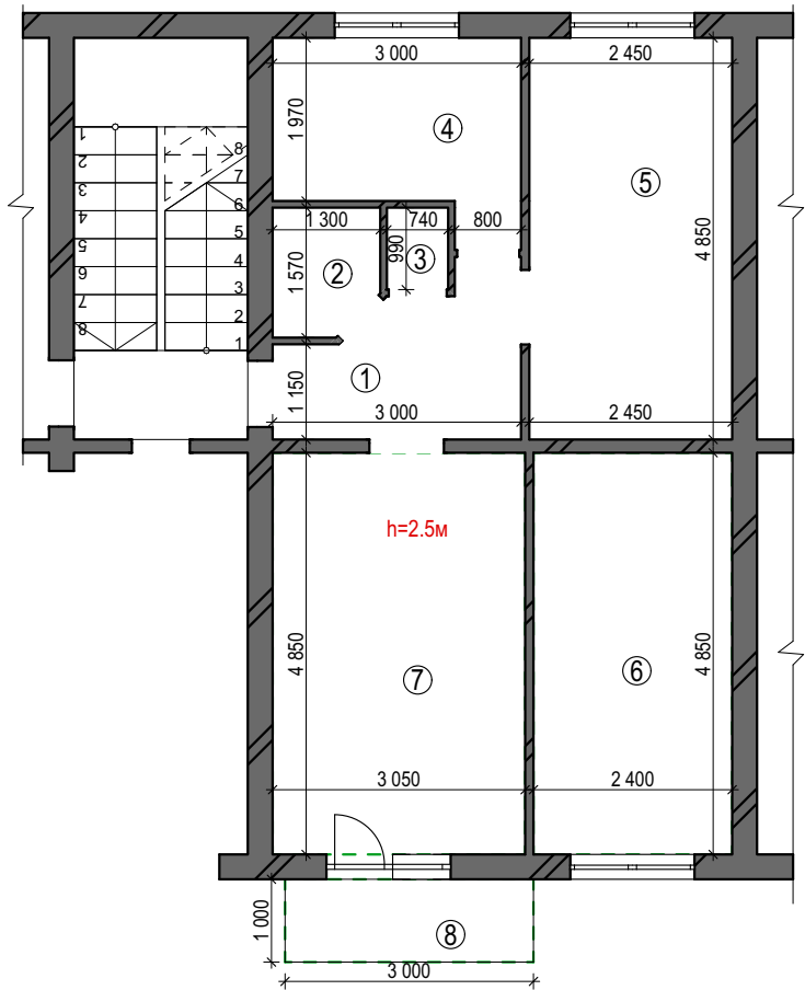
План обмірів М1:100
