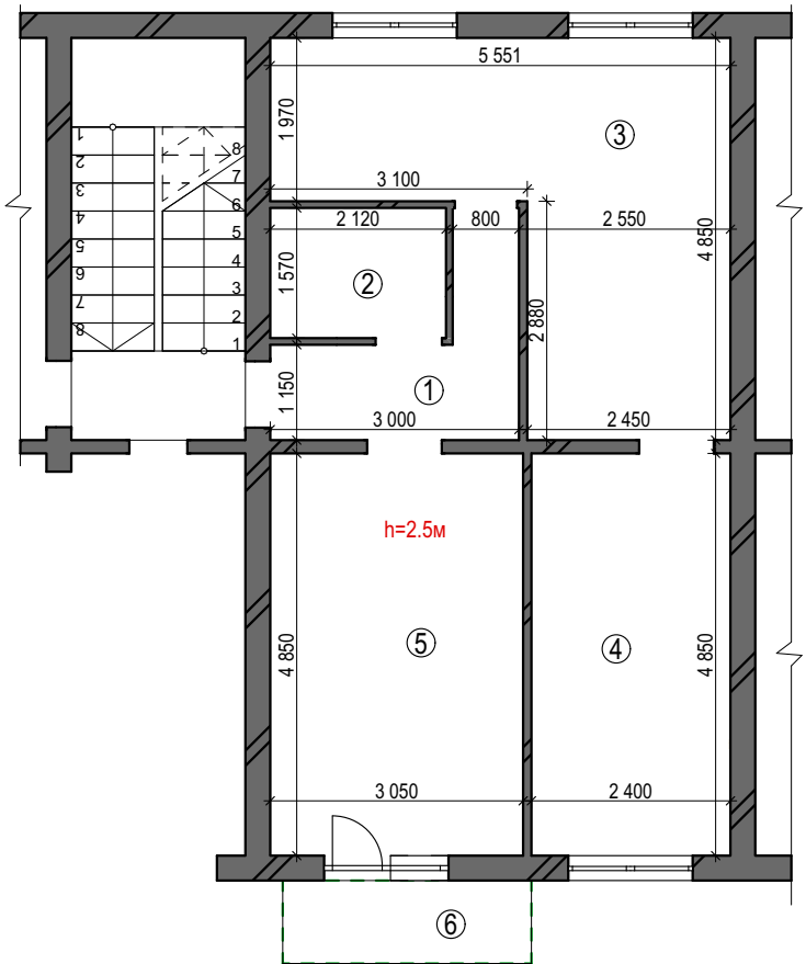
План перепланування М1:100
