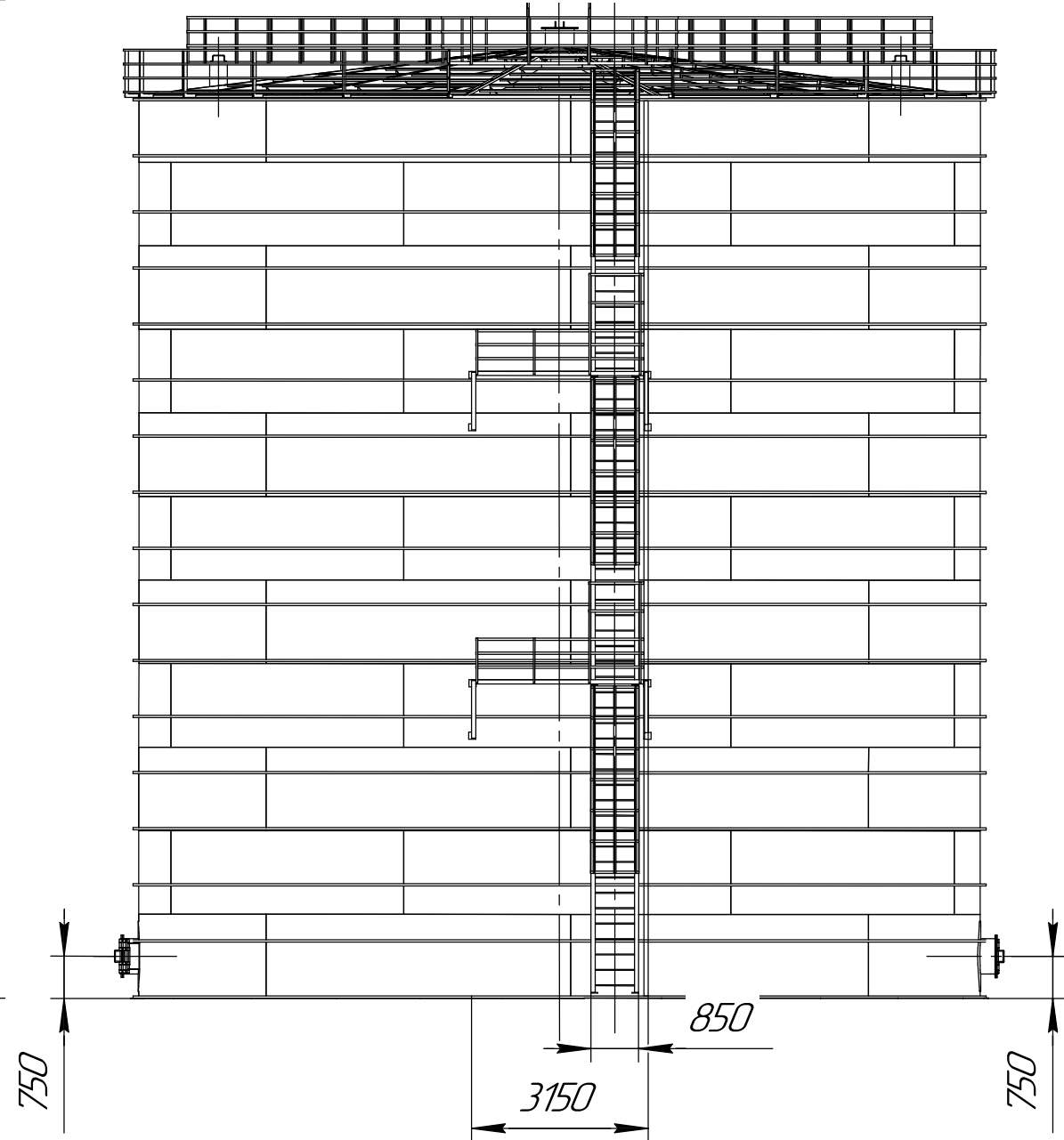
Загальний вид резервуару
