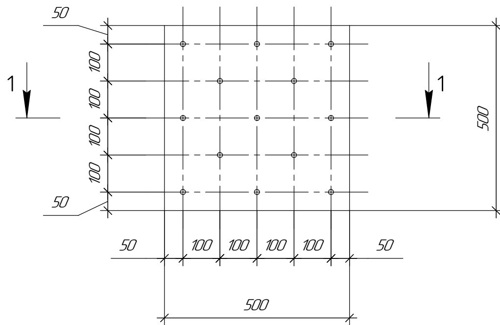
МАКСИМАЛЬНА РІВНОМІРНО- РОЗПОДІЛЕНЕ НАВАНТАЖЕННЯ ПО ВСІЙ ПЛОЩІНІ ДНА РЕЗЕРВУАРУ
