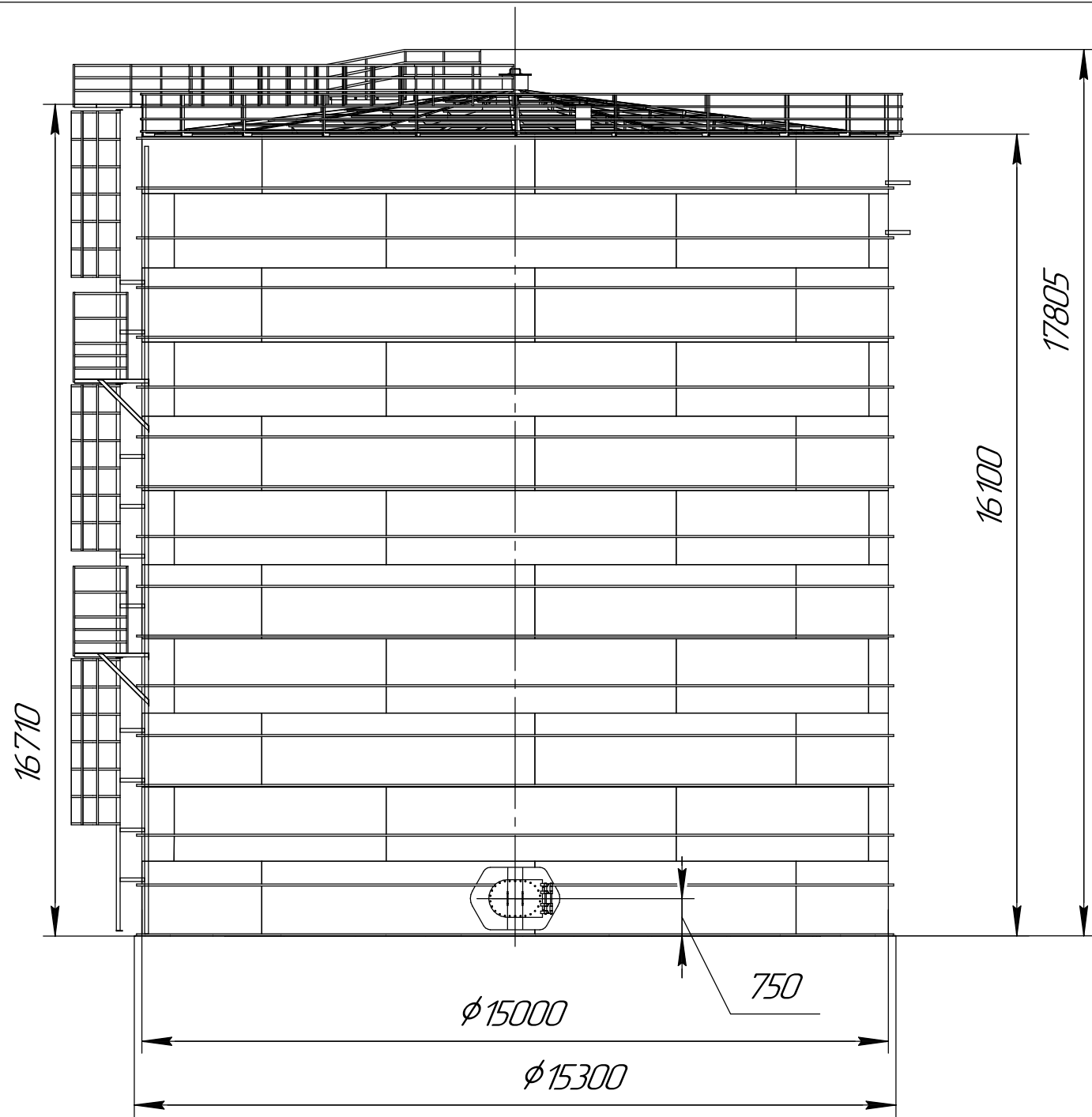
Загальний вид резервуару
