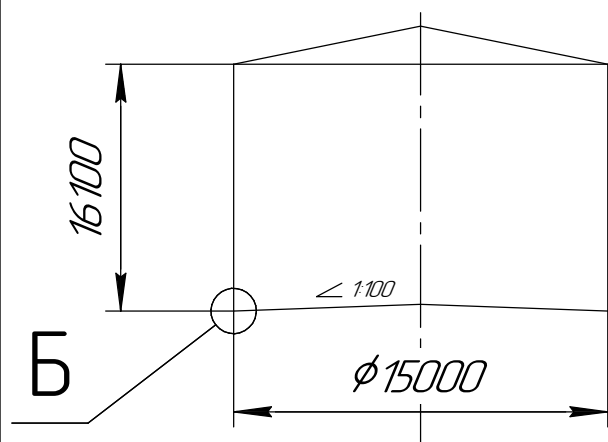
СХЕМА НАВАНТАЖЕНЬ ВІД КОРПУСУ РЕЗЕРВУАРУ ГАБАРИТУ КОРПУСУ РЕЗЕРВУАРУ
