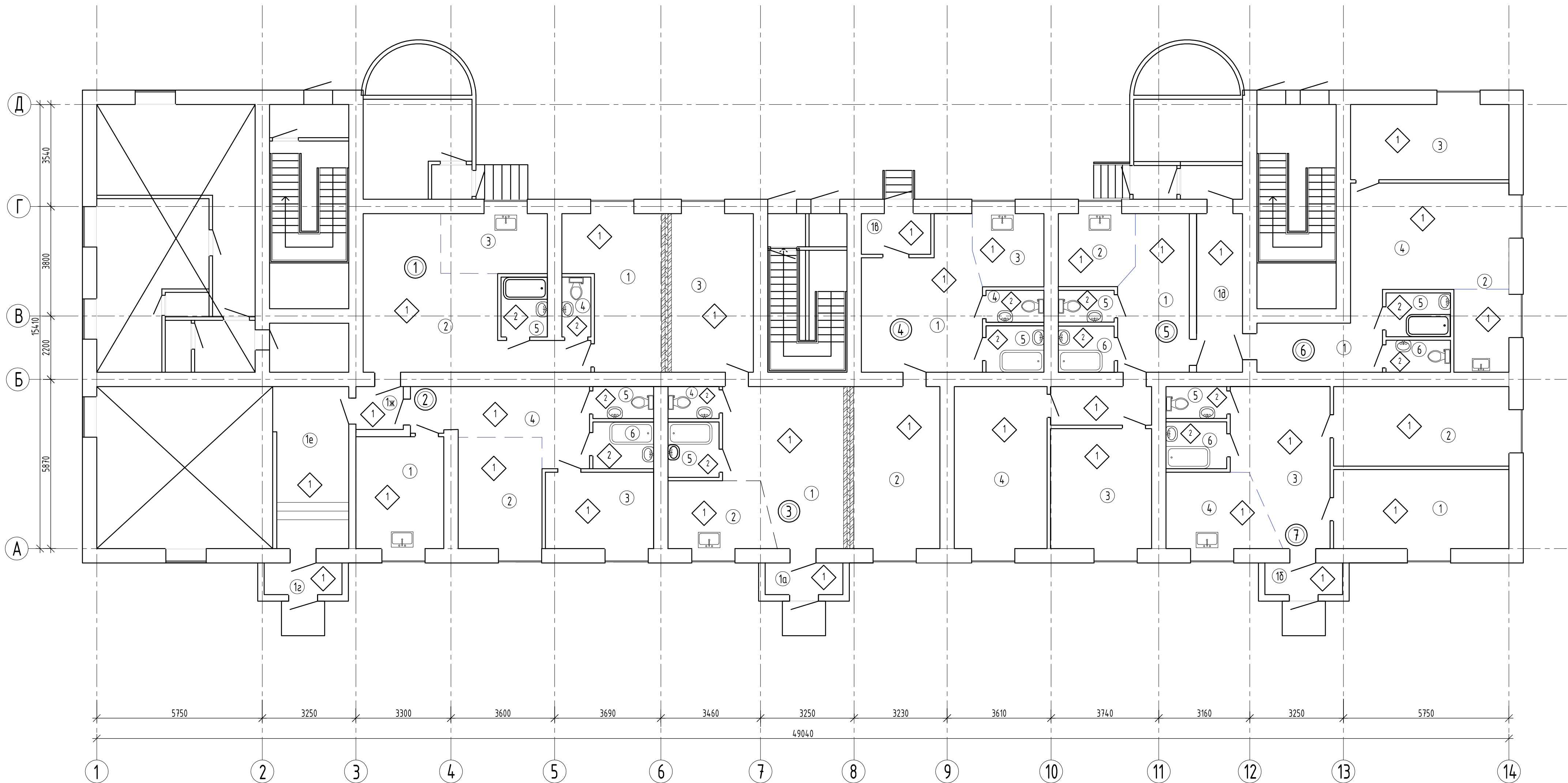
Експлікація оздоблення стель
