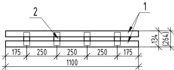
Перетинка Пр-1 (Пр-2)
