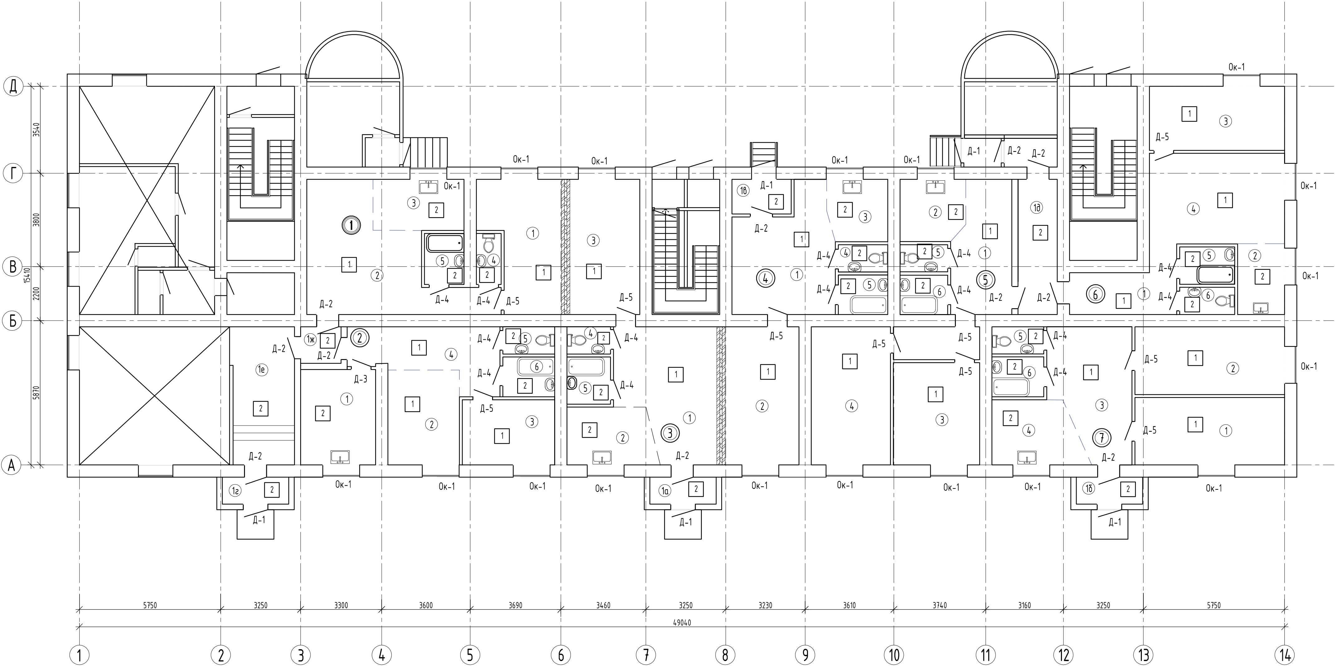
План ремонту підлоги, заміни вікон та дверей
