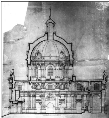
Розріз Домініканського собору у Львові, виконав Кшивоблоцький, керівник Е. Ковач, папір, туш, 72,5 x 61 см.
