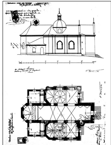
План добудови додаткової нави церкви святого Онуфрія у Львові (1902).
