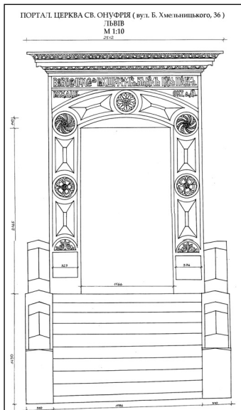
Портал церкви святого Онуфрія у Львові на вулиці Б. Хмельницького, 36. Обмірне креслення 2003 р.
