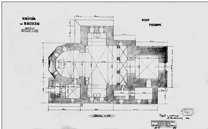
Обмірні креслення костелу в Бушчі, 1910 р.
