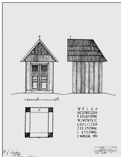
Обмірні креслення каплички на Вулиці Недведзьській, 1931 р.
