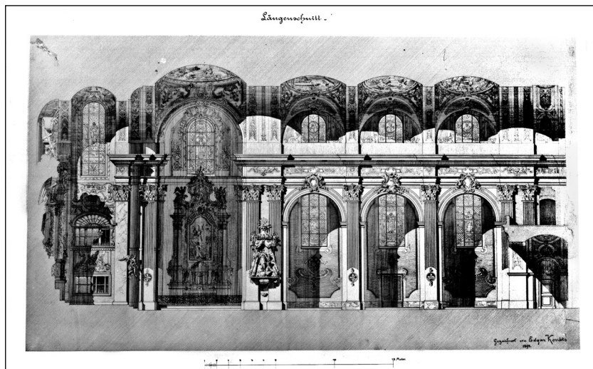
Повздовжній розріз інтер'єру церкви в Маріахілф, графіка Е. Ковача, картон, туш, 54,5 x 80,5 см, 1894 р.
