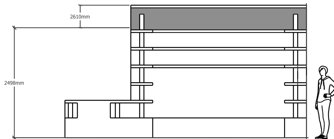
Главный фасад
