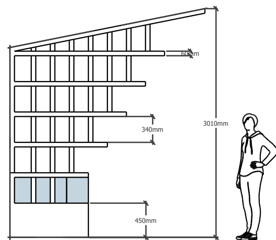
Боковой фасад
