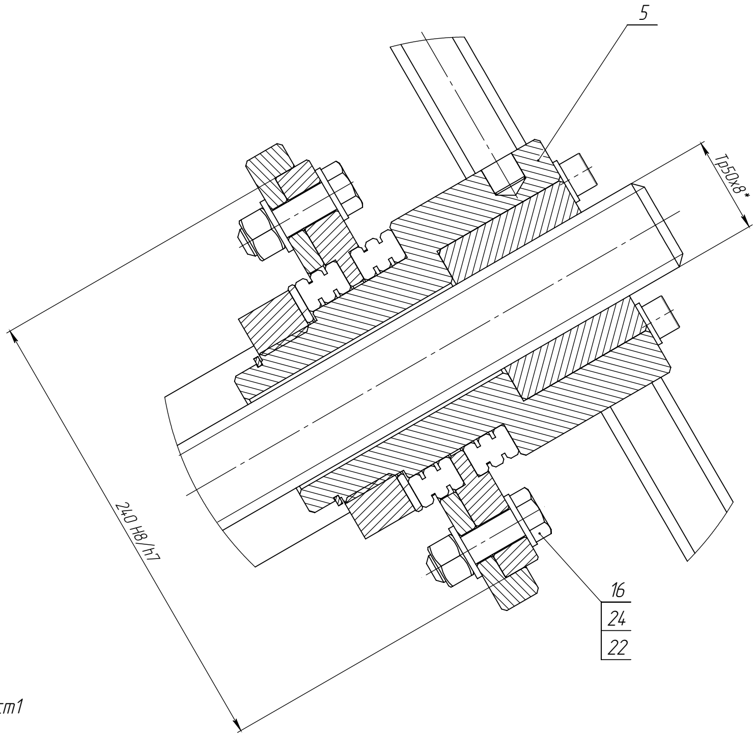
Г (1 : 2)
