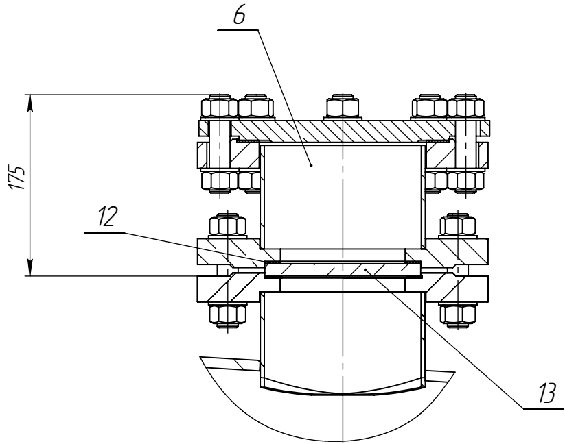
A-A (1 : 5)
