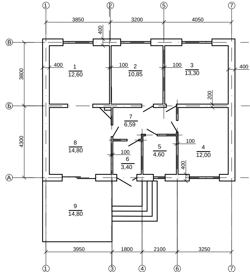
План 1-го поверху на відмітці 0,000
