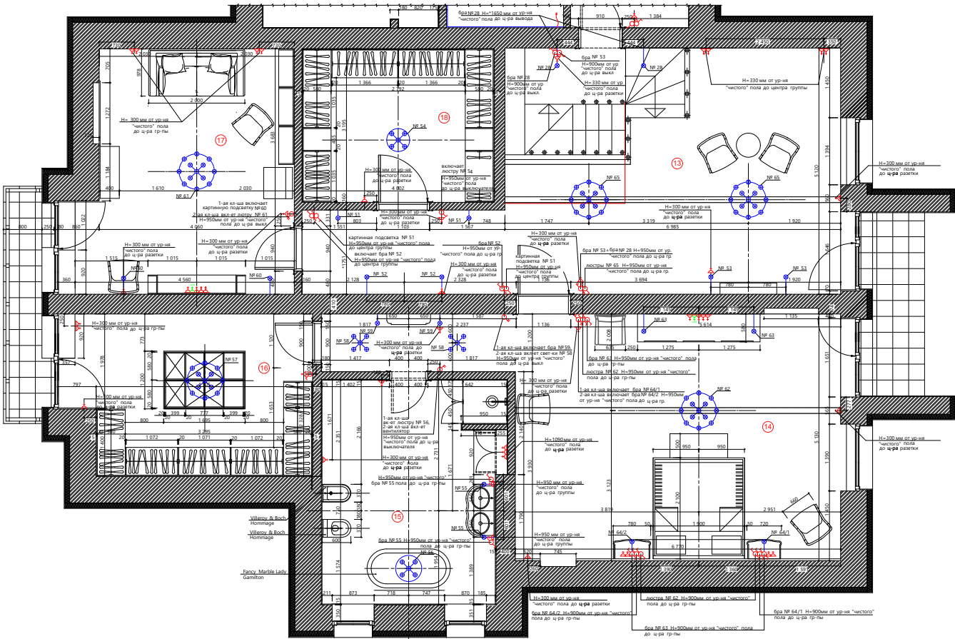
ФРАГМЕНТ ПЛАНУ 1-ГО ПОВЕРХУ
