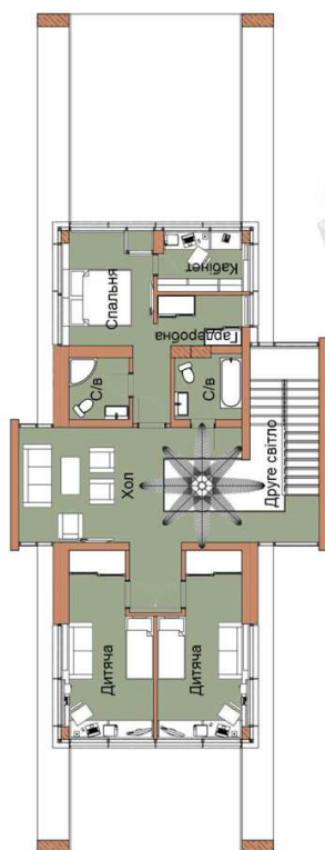
План 2 этажа
