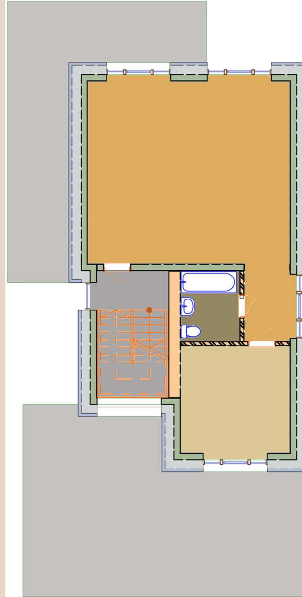
План 2 этажа
