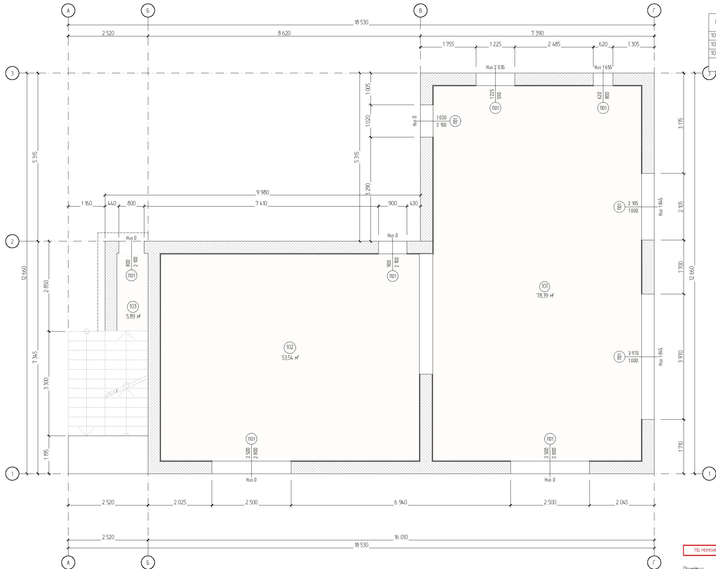
Обмірна експлікація приміщень 1 пов.
