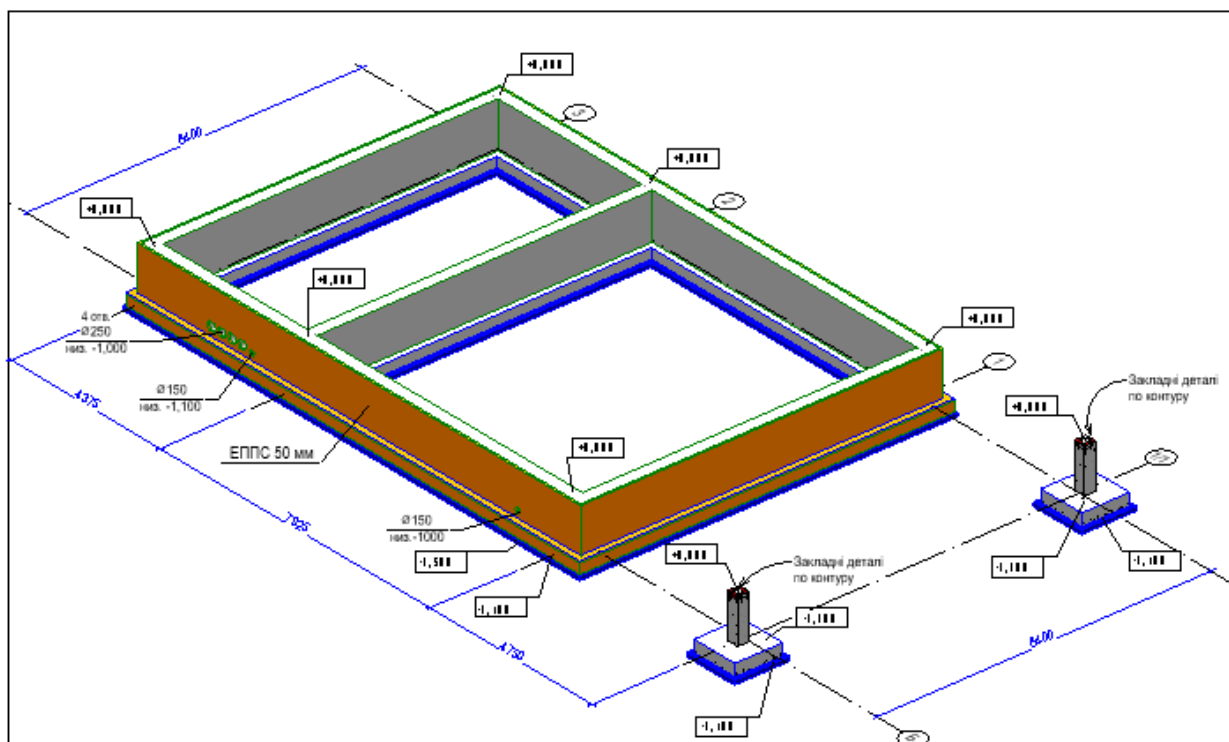
Загальний вигляд фундаменту
