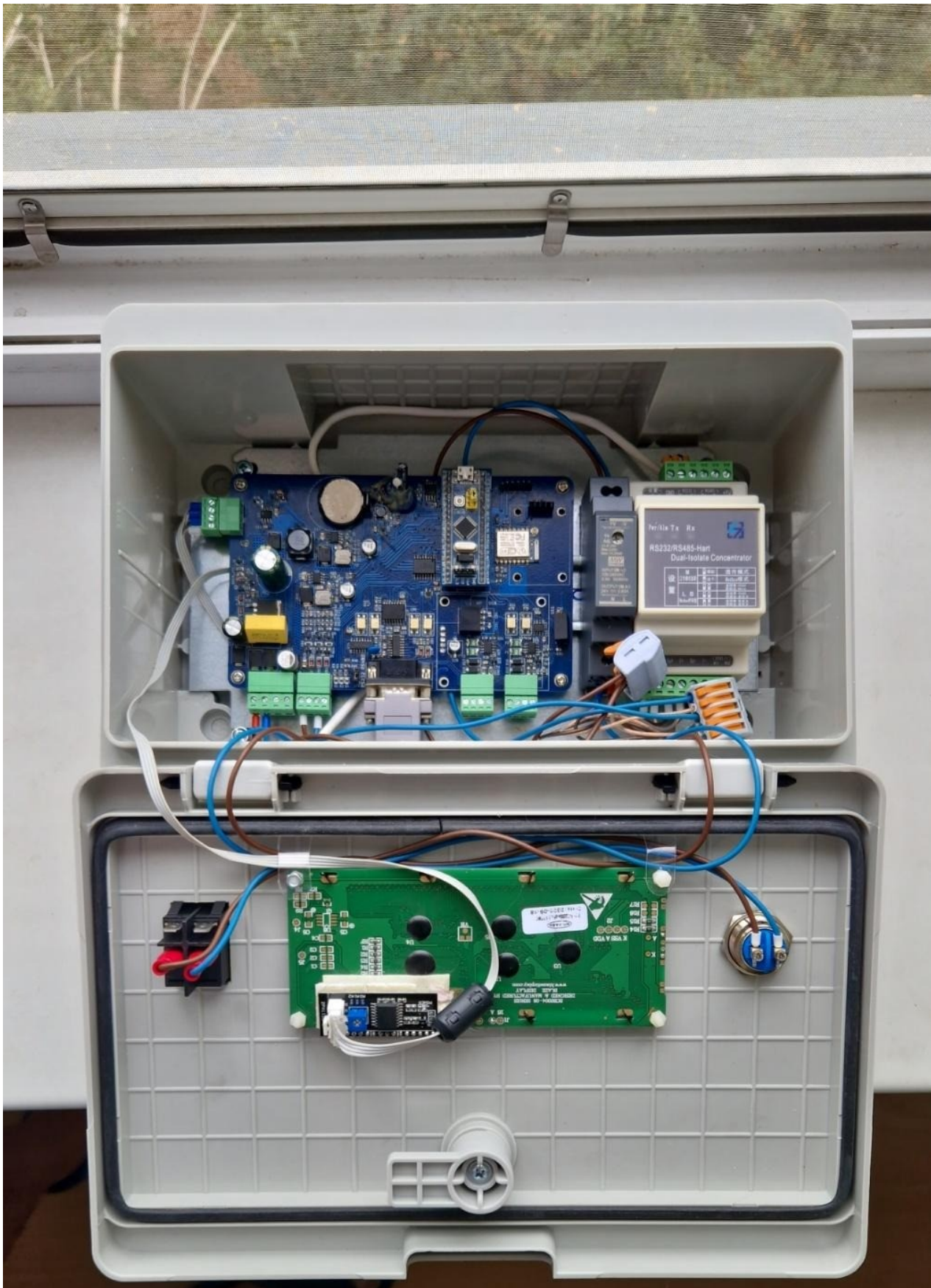
Устройство в сборе
