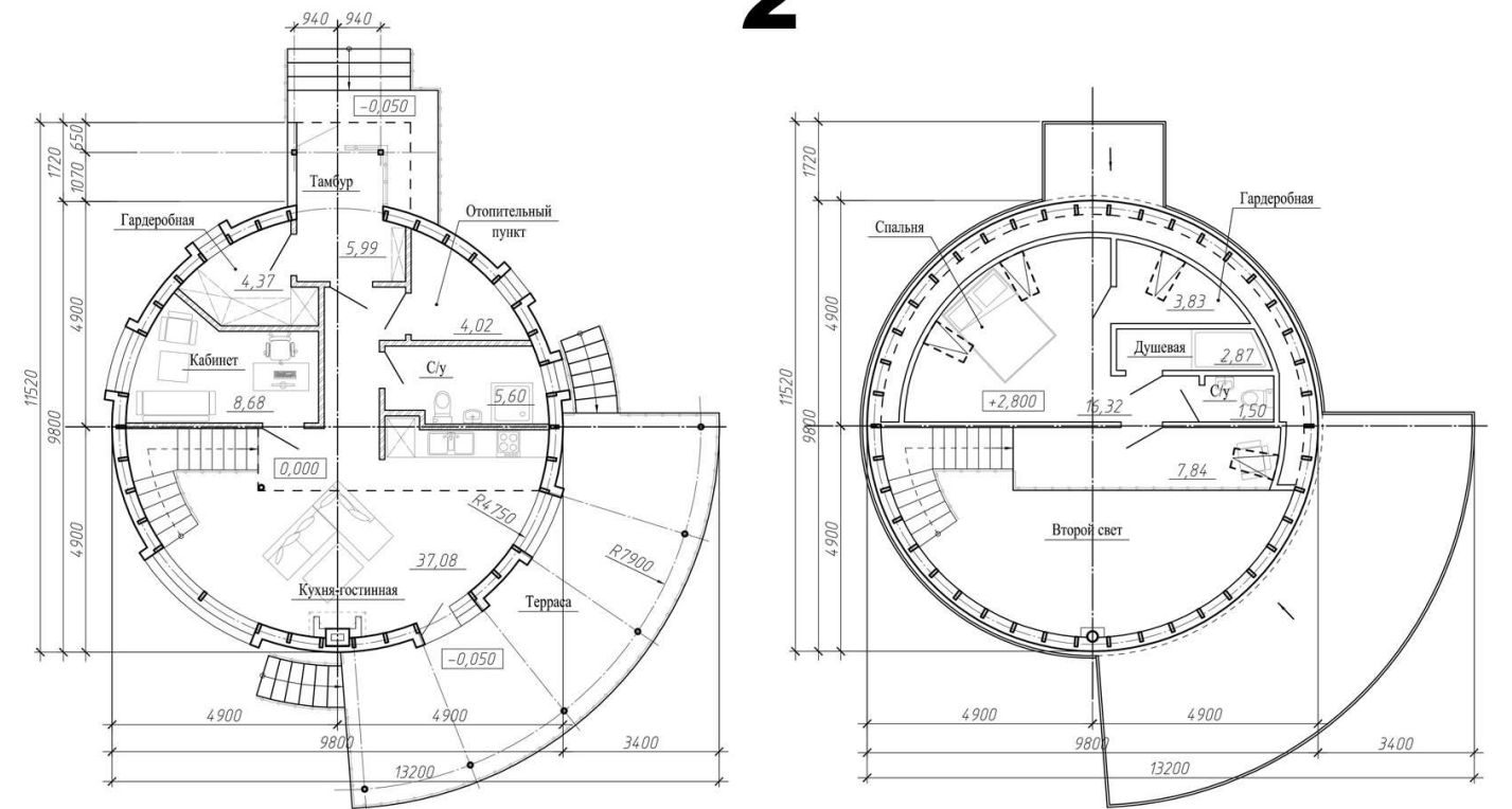
План 2 этажа
