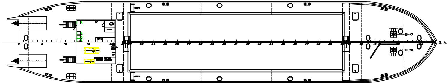
ПЛАН ГЛАВНОЙ ПАЛУБЫ
