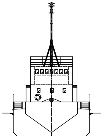
ПРЕДСТАВЛЕННЫЙ ВИД (ВИД НА КОРМУ)
