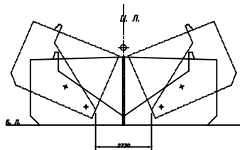
БАРЖА В ОТКРЫТОМ ПОЛОЖЕНИИ
