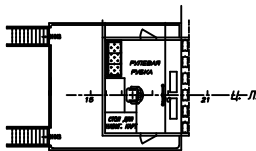
ПЛАН ПАЛУБЫ НАВИГАЦИОННОГО МОСТИКА
