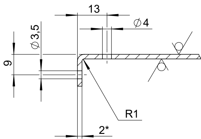
A-A 1:1 2 места
