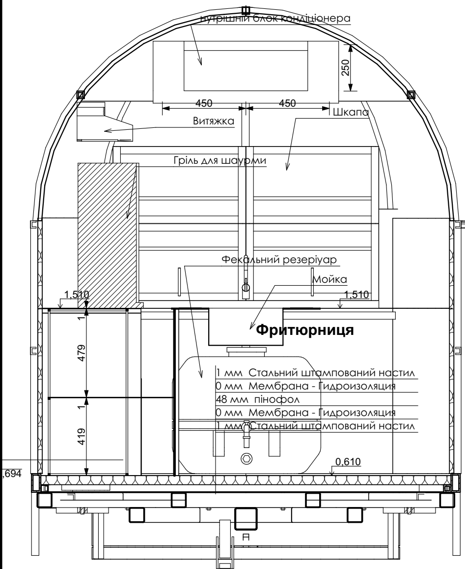
Розріз 3-3
