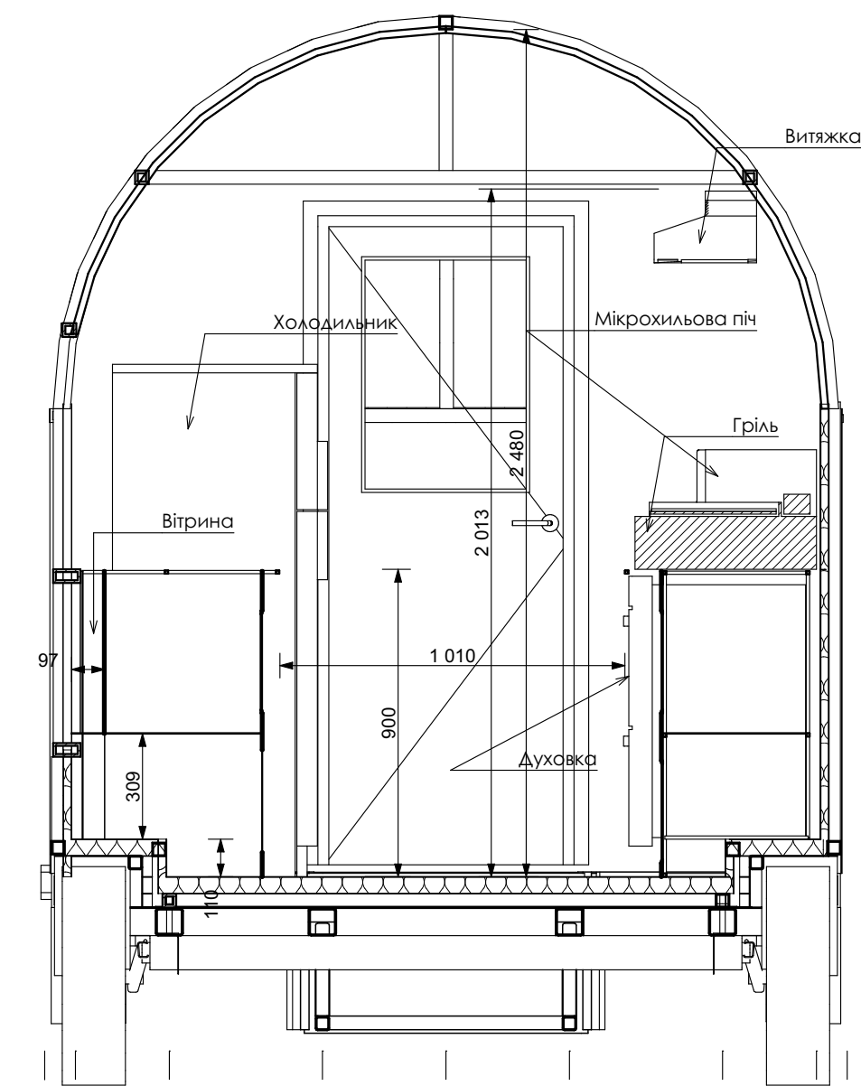
Розріз 5-5
