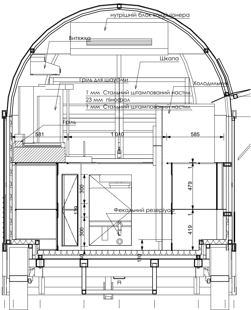
Розріз 4-4
