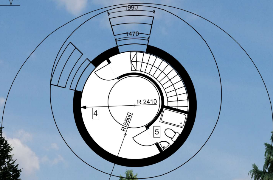
1 План 2-го поверху М1:100
