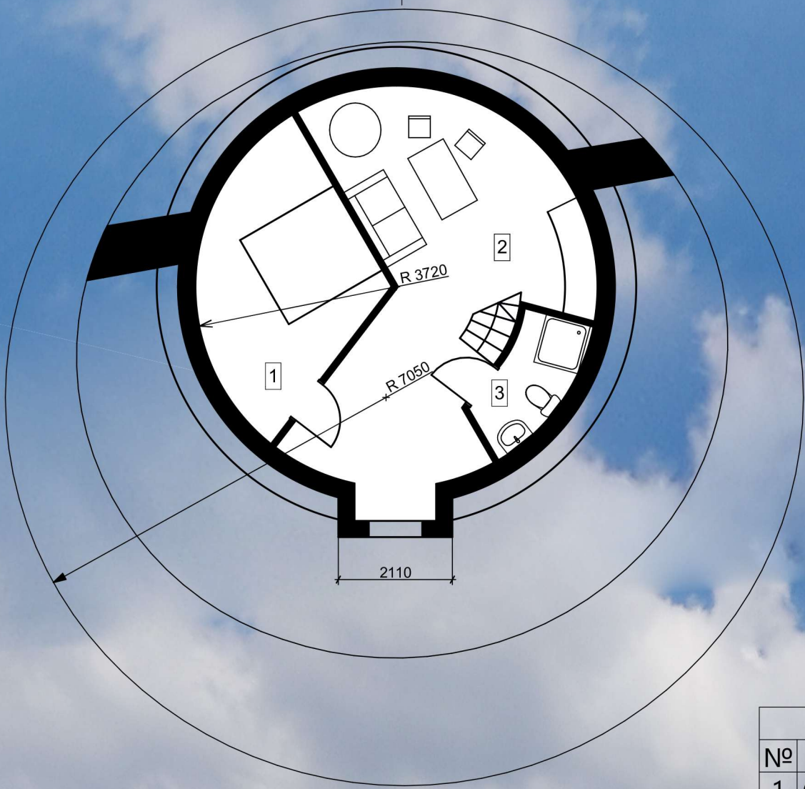
1 План 1-го поверху М1:100
