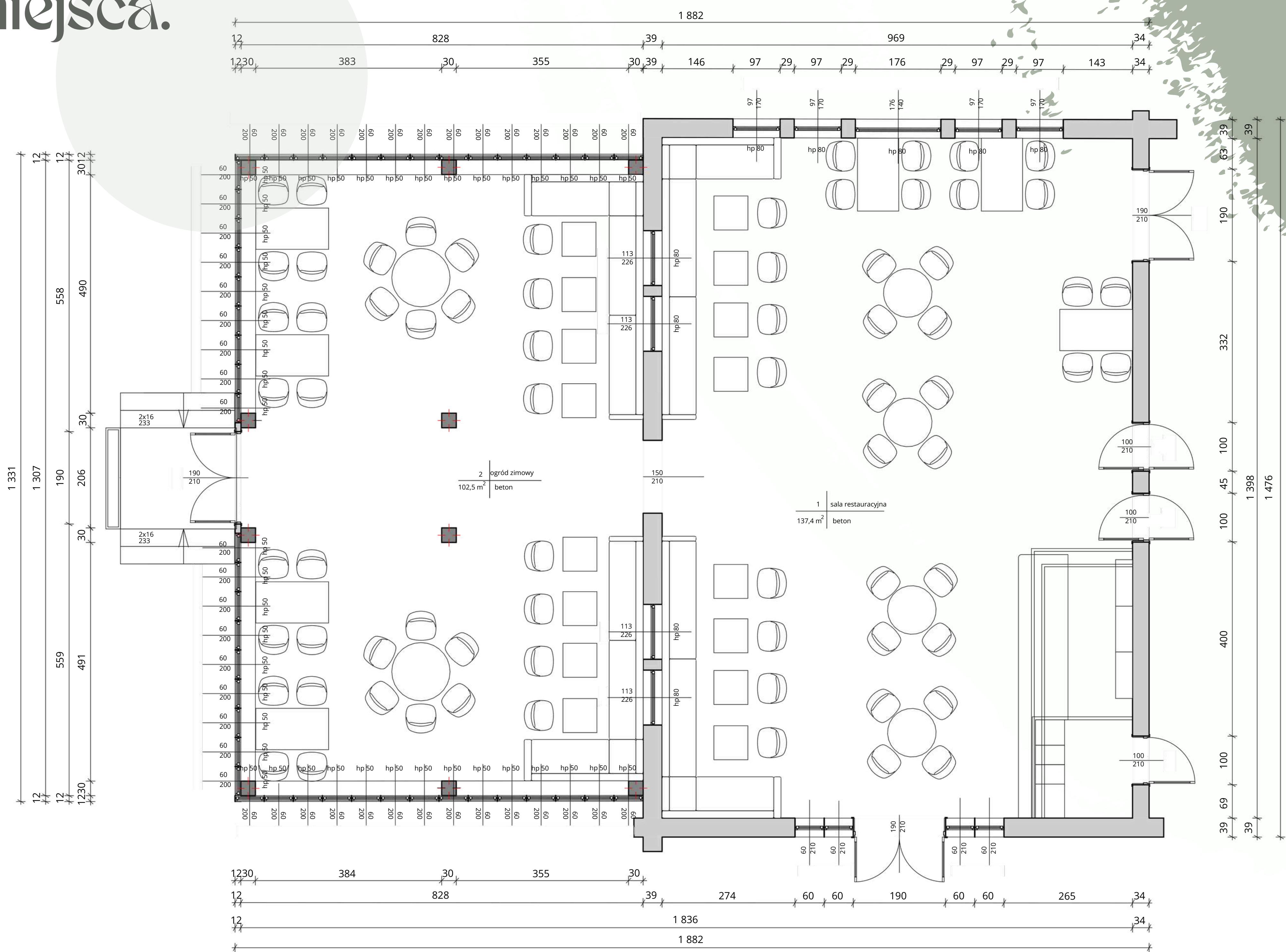
RZUT, SKALA 1:50
